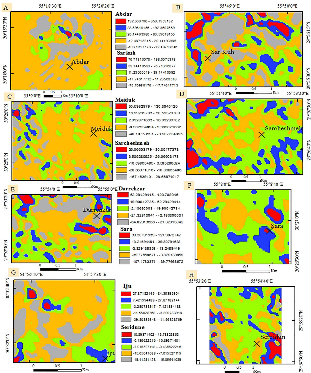
شکل ۵. نقشه فیلتر مشتق اول کانسارهای مطالعاتی. A: ذخیره آبدار، B: ذخیره سرکوه، C: معدن میدوک، D: معدن سرچشمه، E: معدن دره‌زار، F: ذخیره سارا، G: ذخیره ایجو و H: ذخیره سریدون
