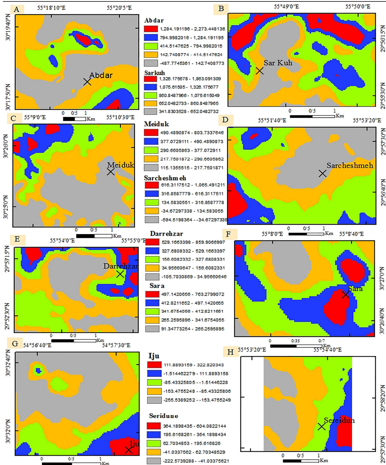
شکل ۴. نقشه‌های تبدیل برگردان به قطب. A: ذخیره آبدار، B: ذخیره سرکوه، C: معدن میدوک، D: معدن سرچشمه، E: معدن دره‌زار، F: ذخیره سارا، G: ذخیره ایجو و H: ذخیره سریدون
