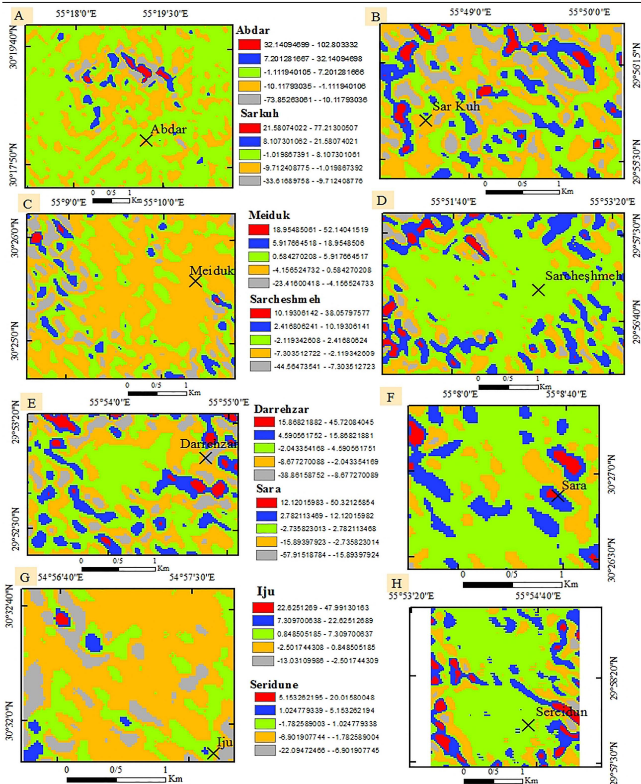
شکل ۶. نقشه فیلتر مشتق دوم کانسارهای مطالعاتی. A: ذخیره آبدار، B: ذخیره سرکوه، C: معدن میدوک، D: معدن سرچشمه، E: معدن دره زار،
