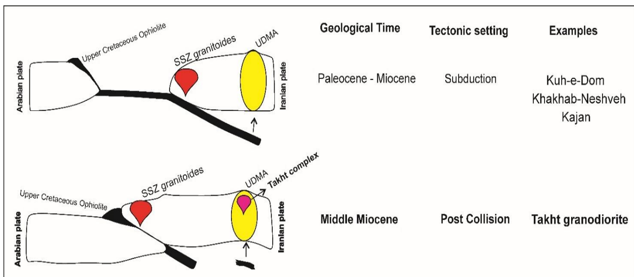
شکل ۱۹. سیر تکامل اقیانوس نئوتتیس و چگونگی تشکیل مجموعه ماگمایی تخت (SSZ: Sanandaj-Sirjan Zone)
