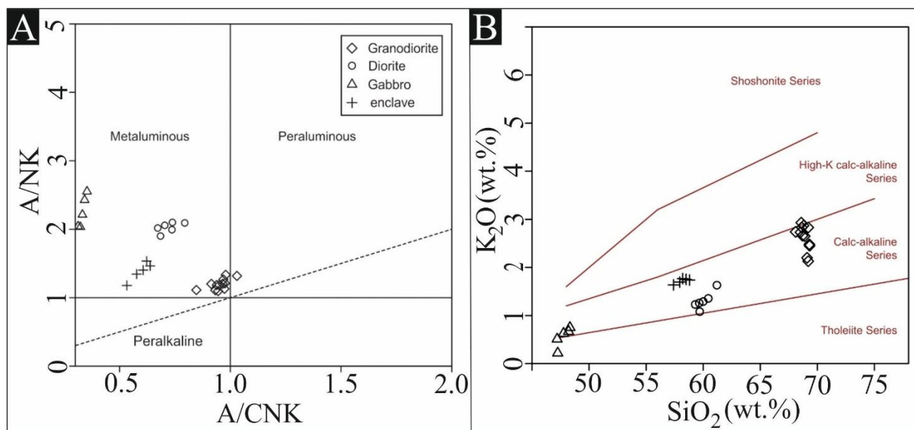
شکل ۸. A: نمودار Al_2O_3/(CaO + Na_2O + K_2O) در برابر Al_2O_3/(Na_2O + K_2O) (نمودار A/CNK-A/NK) (Shand, 1947) نشان‌دهنده ماهیت متالومینوس برای نمونه سنگ‌های درونی منطقه تخت است و B: نمودار K_2O در برابر SiO_2 (Peccerillo and Taylor, 1976) برای تعیین سری ماگمایی نمونه‌ها به کار رفته است که اغلب نمونه‌های منطقه تخت در سری کالک‌آلکان قرار می‌گیرد.
