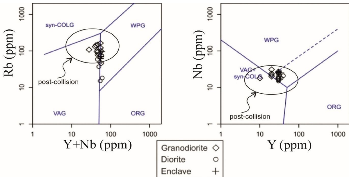
شکل ۱۶. نمودار تعیین محیط زمین‌ساختی نمونه‌های مورد بررسی منطقه تخت (Pearce et al., 1984)، محدوده پس از برخورد از Forster et al. (1997)
