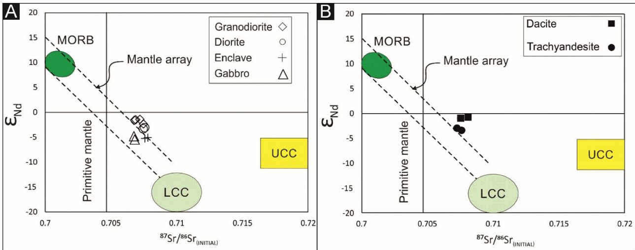
شکل ۱۵. تعیین منشأ با استفاده از نسبت ^{87}\text{Sr}/^{86}\text{Sr} در برابر \epsilon_{\text{Nd}} در منطقه تخت. A: سنگ‌های درونی و B: سنگ‌های بیرونی (UCC: پوسته قاره‌ای بالایی (Taylor and McLennan, 1995)، LCC: پوسته قاره‌ای پایینی (Rudnick and Fountain, 1995))
