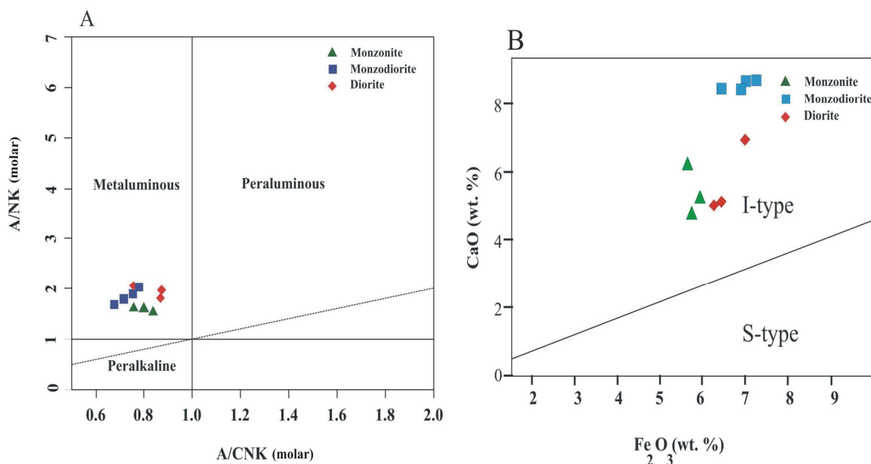
شکل 9. A: نمودار A/NK در برابر A/CNK از سنگ‌های نفوذی منطقه شاه سلطان‌علی (Shand, 1947) و B: نمودار CaO در برابر Fe_2O_3 برای سنگ‌های نفوذی منطقه شاه سلطان‌علی. خط تیره جدا کننده I-type از S-type است (Chappell and White, 2001).
