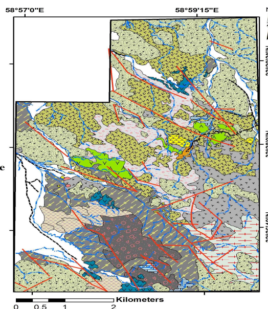
شکل 3. نقشه دگرسانی گستره شاه سلطان‌علی با مقیاس 1:20000
