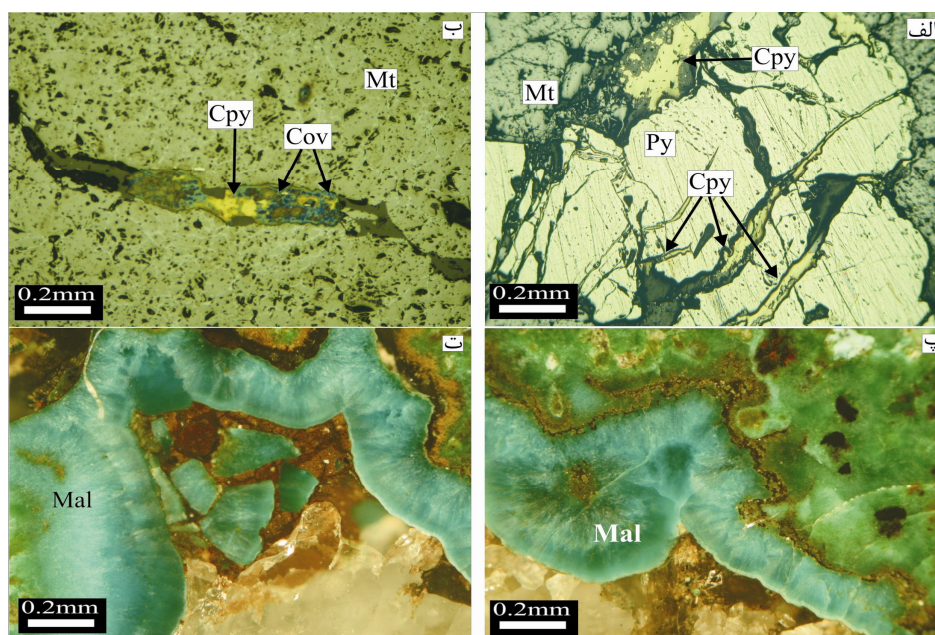
شکل 9. الف) کالکوپیریت با بافت پرکننده شکستگی‌های پیریت، ب) تبدیل کالکوپیریت از حاشیه به کوولیت، پ و ت) مالاکیت با بافت کلوفر-نور (Cpy: کالکوپیریت، Cov: کوولیت، Mal: مالاکیت، Mt: مگنتیت، Py: پیریت). XPL
