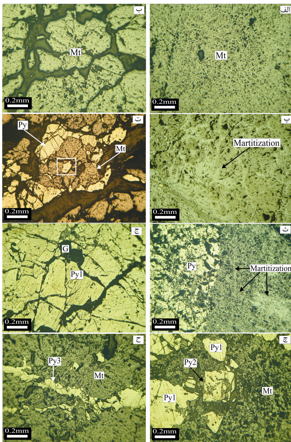
شکل 8. الف) مگنتیت با بافت توده‌ای و ریزدانه، ب) مگنتیت با بافت پرشی (کاتاکلاستی)، پ) مگنتیت با بافت مارتیتی (ت) پیریت‌های جانشین شده توسط مگنتیت، همان‌طور که مشاهده می‌شود پیریت توسط مگنتیت جانشین شده است و به‌صورت جزیره‌ای در وسط باقی‌مانده است و شکل اولیه خود را تا حدودی حفظ کرده است، ث) تصویر میکروسکوپی از بافت مارتیتی در کانسار آهن ظفرآباد، همان‌طور که مشاهده می‌شود مگنتیت به هماتیت تبدیل شده است در صورتی‌که پیریت‌ها کاملاً دست‌نخورده باقی‌مانده‌اند، ج) تصویر میکروسکوپی از پیریت‌های نوع اول (Py1) با بافت کاتاکلاستی، چ) تصویر میکروسکوپی از پیریت‌های خود شکل نوع دوم (Py2) در کنار پیریت‌های بی‌شکل نوع اول (Py1) که تا حدودی توسط مگنتیت جانشین شده‌اند، ح) پیریت‌های رگه‌ای نوع سوم (Py3) که به‌صورت رگه‌چه‌هایی مگنتیت را قطع کرده است - نور PPL، PPL: مگنتیت، Py: پیریت، G: گانگ.
