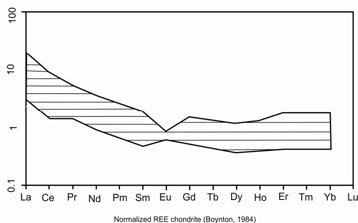
شکل 12. الگوی توزیع عناصر نادر خاکی در نمونه‌های کانسنگ مگنتیتی ظفرآباد نرمالیزه شده با کندریت [23].
