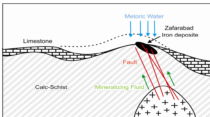
شکل 16. مدل پیشنهادی تشکیل کانسار آهن ظفرآباد.
