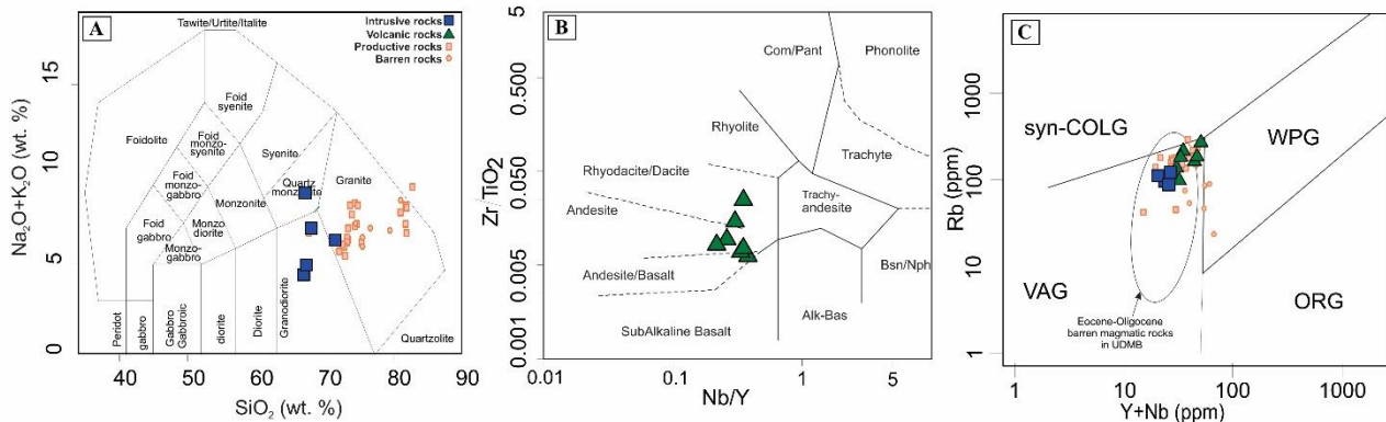
شکل ۴. طبقه‌بندی زمین‌شیمیایی A: Na_2O+K_2O در برابر SiO_2 (Middlemost, 1994) برای توده‌های نفوذی و B: Zr/TiO_2 در برابر Nb/Y برای سنگ‌های آتشفشانی (Winchester and Floyd, 1977) و C: موقعیت سنگ‌های آذرین لاله‌زار در نمودار Rb vs. Y+Nb (Pearce et al., 1984)
