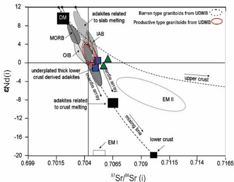
شکل ۷. نمودار \epsilon_{Nd}(i) اولیه نسبت به ^{87}Sr/^{86}Sr(i) برای سنگ‌های آذرین لاله‌زار
