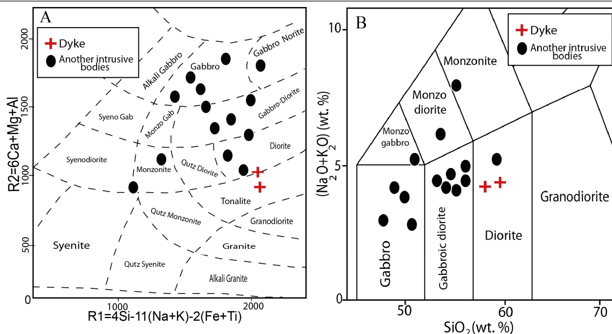
شکل ۶. A: طبقه‌بندی ژئوشیمیایی و نام‌گذاری سنگ‌های آذرین درونی تاریک‌دره بر اساس نمودار R2- R1 (De la Roche et al., 1980) و B: طبقه‌بندی با استفاده از نمودار مجموع \text{Na}_2\text{O} + \text{K}_2\text{O} در مقابل \text{SiO}_2 (Middlemost, 1985)
