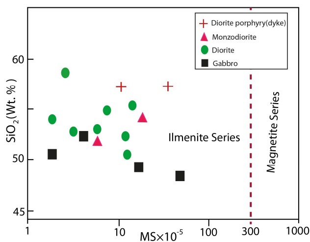
شکل ۱۰. تغییرات \text{SiO}_2 در مقابل پذیرفتاری مغناطیسی برای سنگ‌های نفوذی منطقه تاریک‌دره
