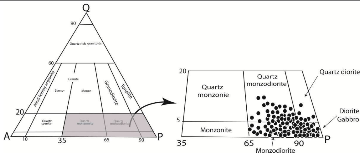
شکل ۴. بررسی مودال سنگ‌های آذرین درونی منطقه تاریک‌دره در نمودار اشتراک‌ایزن (Streckeisen, 1974) نشان می‌دهد که سنگ‌ها ترکیبی حدواسط دارند.
