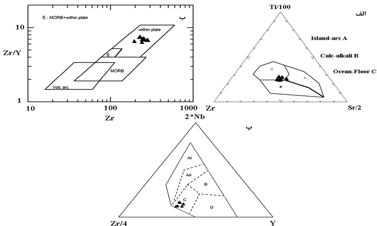
شکل 12. الف) ترسیم نمونه‌ها در نمودار Zr-Ti/100-Sr/2 [27]، ب) ترسیم نمونه‌ها در نمودار Zr/Y-Zr [28] در محدوده درون صفحه‌ای قرار می‌گیرند، پ) ترسیم نمونه‌ها در نمودار Zr/4-Nb*2-Y [29] محدوده تولیتهای داخل صفحه‌ای را نشان می‌دهد.
