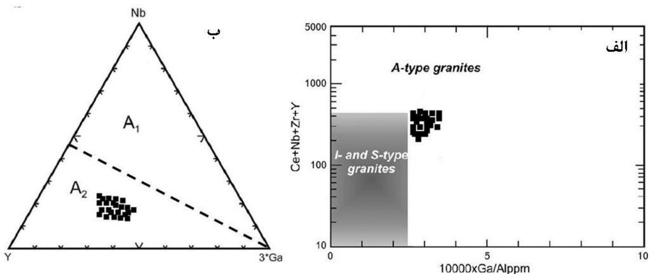
شکل 13. الف) در نمودار تفکیک گرانیت‌های Ce+Nb+Zr+Y در مقابل 10,000 \times Ga/Al ، نمونه‌های مطالعه‌شده در قلمرو تیپ A قرار می‌گیرند [33]، ب) در نمودار سه‌تایی Y-Nb-3 \times Ga ، نمونه‌ها در قلمرو A_2 قرار می‌گیرند [34].
