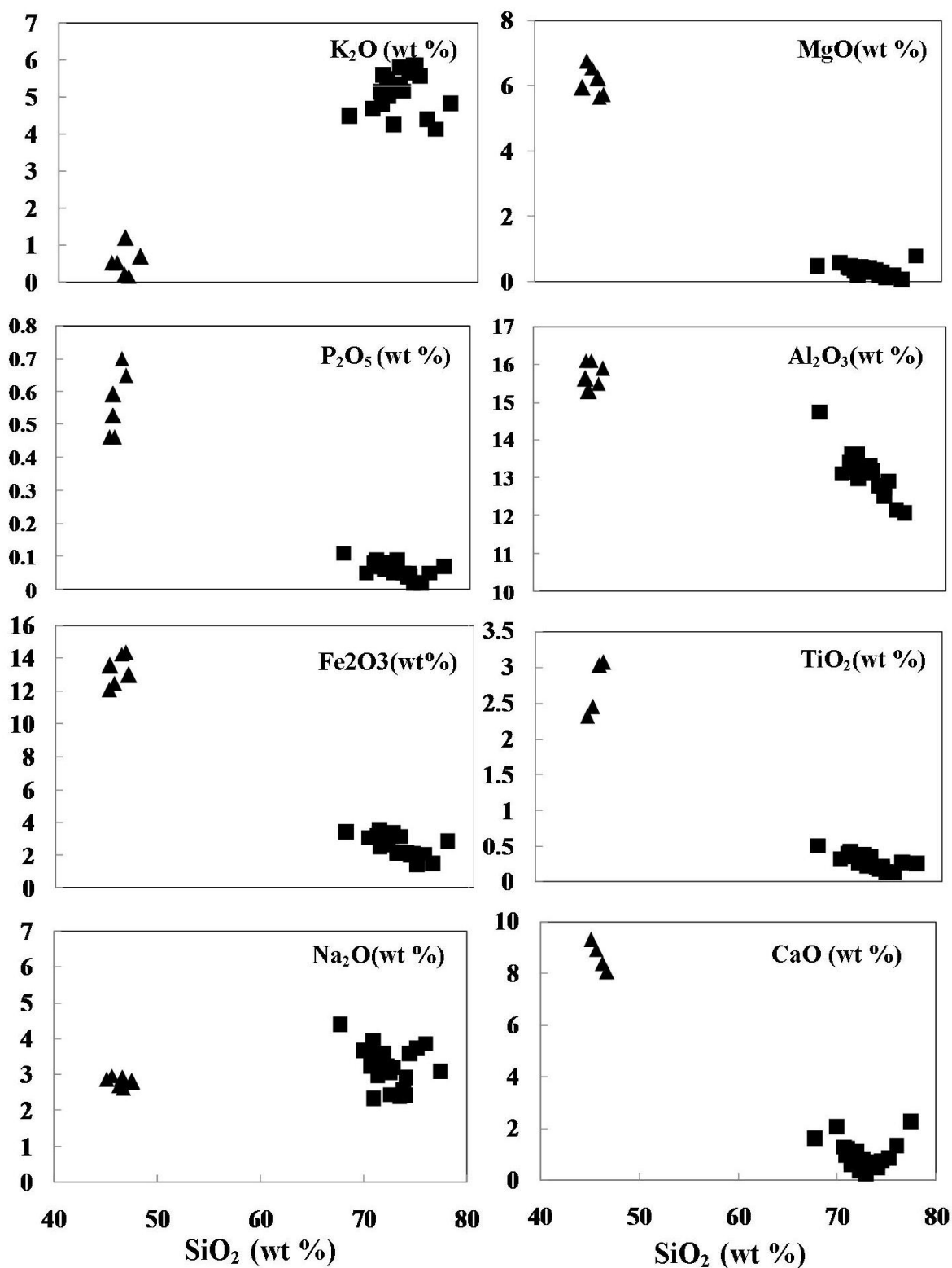
شکل 9. ترسیم تغییرات اکسیدها در مقابل سیلیس در نمودار [14]
