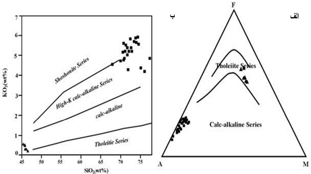
شکل 7. الف) نمونه‌های گرانیتوئیدی و بازیک در نمودار AFM [11]، ب) در نمودار K_2O در مقابل SiO_2 نمونه‌های اسیدی و گابرو به ترتیب در قلمرو کالکوالکالن غنی از پتاسیم و تولیتیته قرار می‌گیرند [12].
