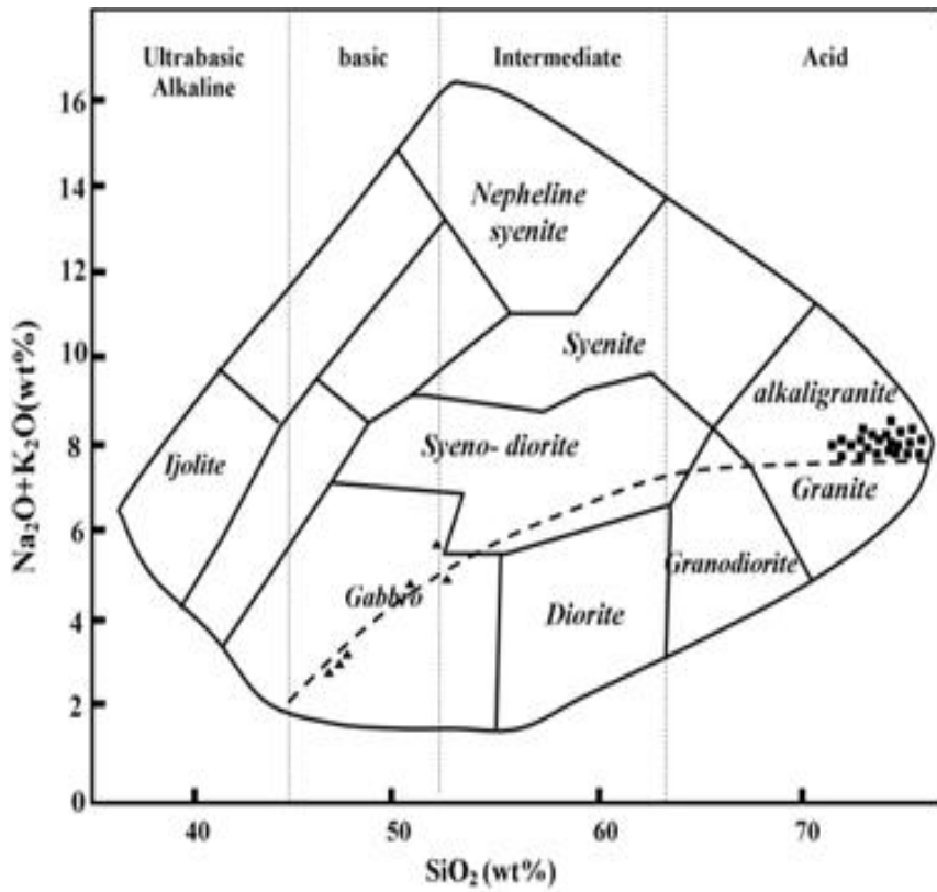
شکل 6. نمودار تغییرات Na_2O+K_2O در مقابل SiO_2 نمونه‌های فلسیک در محدوده آلکالی‌گرانیته و نمونه‌های مافیک در محدوده گابرو پلات می‌شوند [9 و 10]. مربع = فلسیک و مثلث = مافیک
