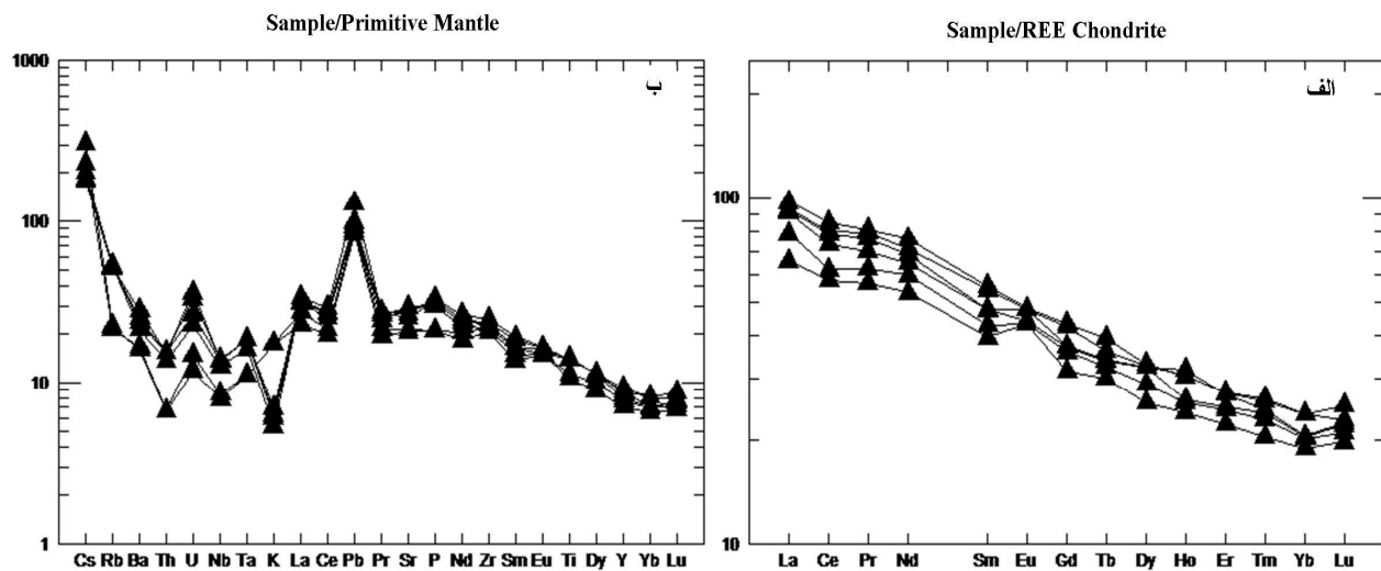
شکل 10. الف) تغییرات فراوانی REE بهنجار شده گابروها نسبت به کندریت [15]، ب) تغییرات فراوانی عناصر اصلی و کمیاب بهنجار شده نسبت به گوشته اولیه [15].
