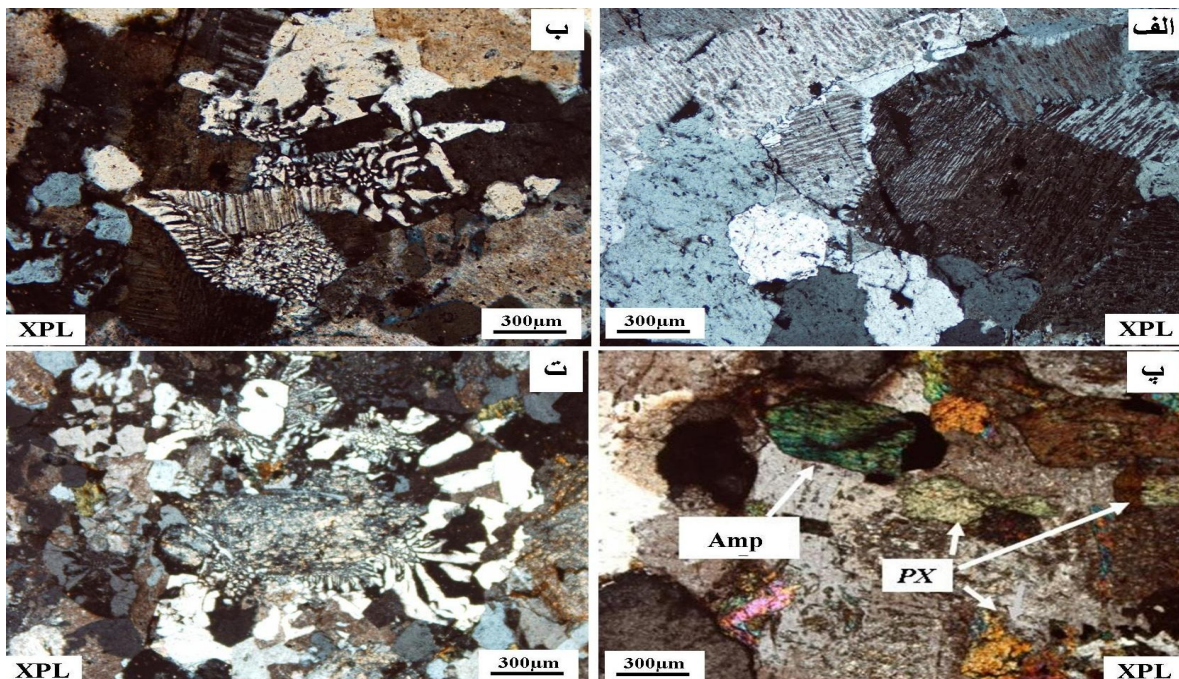
شکل 4. الف) بافت پرتیتی، ب) بافت میکروگرافیکی، پ) بافت گرانولار با کانیهای امفیبول و بقایایی از پیروکسن، ت) بافت گرانوفیری اطراف ارتوز در گرانیت‌ها. (نور XPL) (آمفیبول=Amp، پیروکسن=PX) [49]
