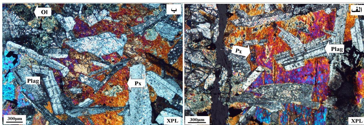
شکل 5. الف و ب) بافت گرانولار دانه‌درشت و حضور کانیه‌های پلاژیوکلاز، پیروکسن در گابروها (نور XPL) (آمفیبول=Amp، پیروکسن=Px، پلاژیوکلاز=Pl) [49]
