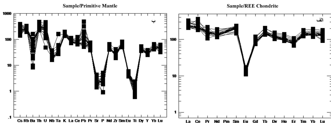
شکل 11. الف) تغییرات فراوانی REE بهنجار شده گرانیت‌ها نسبت به کندریت [15]، ب) تغییرات فراوانی عناصر اصلی و کمیاب بهنجار شده نسبت به گوشته اولیه [15].
