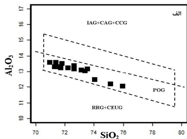
شکل 15. الف) در نمودار تفکیک محیط تکتونیکی، گرانیت‌های مورد مطالعه در محدوده پس از کوهزایی قرار می‌گیرند [12]. ب) در نمودار تعیین محیط زمین‌ساختی نمونه‌ها در محدوده حاشیه قاره‌ای قرار می‌گیرند [38].
