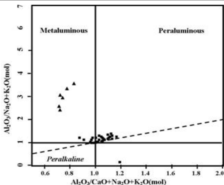
شکل 8. در نمودار شاخص اشباع‌شدگی از آلومینیم (ASI)، نمونه‌های فلسیک در محدوده پرآلومینوس تا متآلومینوس قرار می‌گیرند و نمونه‌های مافیک در محدوده متآلومینوس واقع می‌شوند [13].
