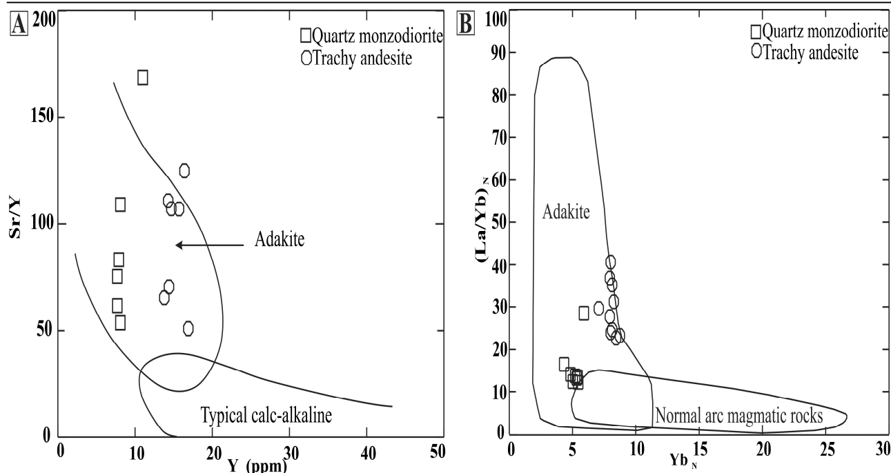
شکل ۹. نمودارهای ژئوشیمیایی تفکیک مذاب‌های حاصل از اسلب فرورونده از ماگماهای کالک‌آلکالن و موقعیت کوارتز مونزودیوریت پورفیری و دایک‌های تراکی‌آندزیت جنوب‌غرب جندق در؛ A: نمودار Y-Sr/Y (Defant and Drummond, 1990) و B: نمودار مقادیر بهنجارشده Yb_N - (La/Yb)_N (Martin, 1999)
