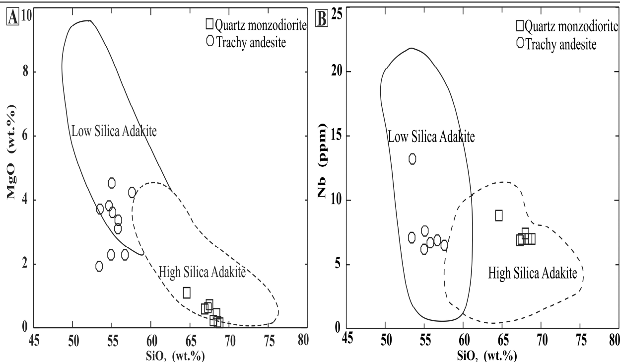
شکل ۱۰. نمودارهای ژئوشیمیایی تفکیک آداکیت‌های پر سیلیس از آداکیت‌های کم سیلیس و موقعیت کوارتز مونزودیوریت پورفیری و دایک‌های تراکی‌آندزیتی جنوب‌غرب جندق در A: نمودار \text{SiO}_2\text{-MgO} (Martin et al., 2005) و B: نمودار \text{SiO}_2\text{-Nb} (Martin et al., 2005)
