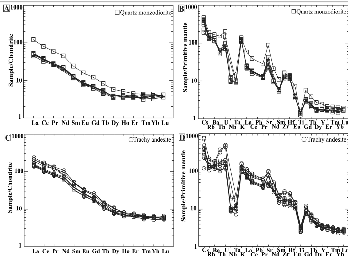
شکل ۸. نمودارهای بهنجارسازی کوارتز مونزودیوریت پورفیری و دایک‌های تراکی‌آندزیتی جنوب غرب جندق در؛ A: الگوی بهنجارسازی عناصر نادر خاکی کوارتز مونزودیوریت‌ها نسبت به ترکیب کندریت، B: نمودار چند عنصری بهنجارشده کوارتز مونزودیوریت‌ها نسبت به ترکیب گوشته اولیه، C: الگوی بهنجارسازی عناصر نادر خاکی دایک‌های تراکی‌آندزیتی نسبت به ترکیب کندریت و D: نمودار چند عنصری بهنجارشده دایک‌های تراکی‌آندزیتی نسبت به ترکیب گوشته اولیه. (داده‌های کندریت برگرفته از مک‌دوناف و سان (McDonough and Sun, 1995) و داده‌های گوشته اولیه برگرفته از سان و مک‌دوناف (Sun and McDonough, 1989))
