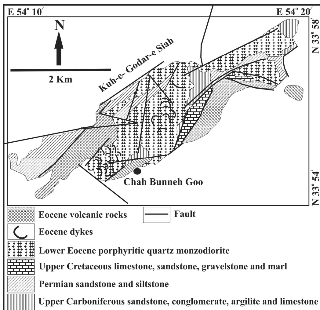
شکل ۳. نقشه زمین‌شناسی ساده‌شده از کوه گدارسیاه (جنوب‌غرب جندق) و موقعیت کوارتز مونزودیوریت پورفیری و دایک‌های قطع‌کننده آن
