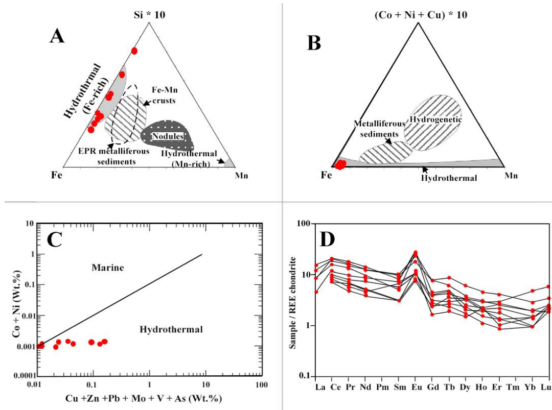
شکل 10. A: نمودار سه‌تایی Fe-Mn-(Si*10) طبقه‌بندی کانسارهای آهن - منگنز (Toth, 1980; Nath et al. 1997). B: نمودار سه‌تایی (Co + Ni + Cu)*10-Fe-Mn طبقه‌بندی کانسارهای آهن - منگنز (Bonatti et al., 1972; Toth 1980). C: نمودار دوتایی Ni+Co در مقابل Cu+Zn+Pb+Mo+V+As طبقه‌بندی کانسارهای آهن - منگنز (Crerar et al., 1982). D: نمودار عنکبوتی عناصر نادر خاکی محدوده اکتشافی فرزانه نرمالیزه شده به کندریت (Boynton 1984).
