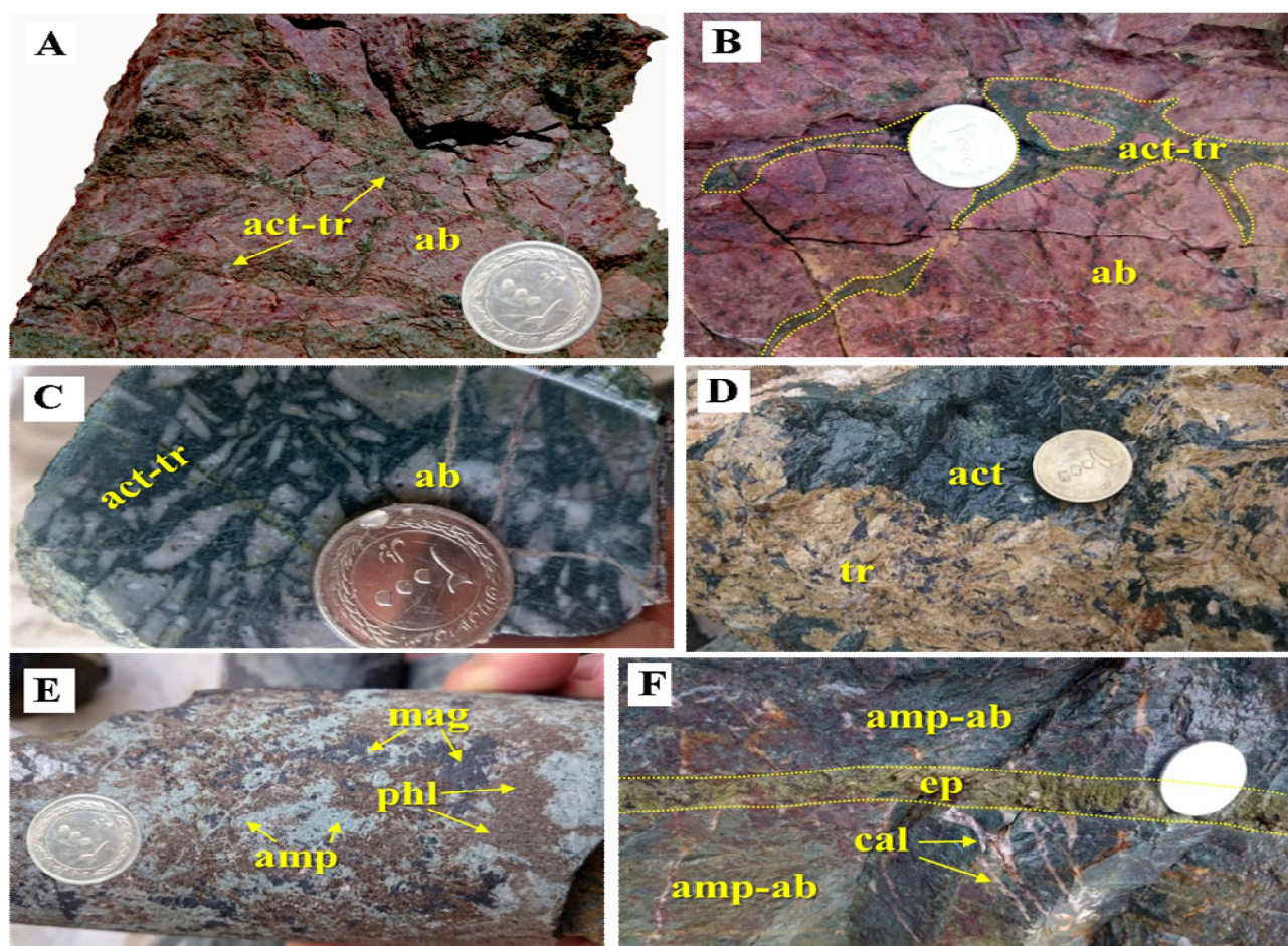
شکل ۴. انواع سنگ‌های دگرنهادی در کانسار ساغند، A: آلپیتیت با ظاهری پرشی در دگرنهاد آمفیبولی، B: رگه‌چه‌های دگرنهاد آمفیبولی درون آلپیتیت، C: آلپیتیت سفیدرنگ با بافت پورفیروکلاستیک در زمینه‌ای از دگرنهاد آمفیبولی، D: دگرنهاد ترمولیتی-اکتینولیتی، E: بلورهای فلوگوپیت و مگنتیت به صورت رونهشتی در دگرنهاد آمفیبولی و F: رگه‌چه اپیدوت که دگرنهاد آمفیبولی-آلپیتی را قطع کرده است. ab: آلپیتیت، act-tr: اکتینولیت-ترمولیت، ترمولیت، mag: مگنتیت، phl: فلوگوپیت، amp: آمفیبول، ep: اپیدوت، علایم اختصاری کانی‌ها بر اساس ویتنی و اوانز (Whitney and Evans, 2010)
