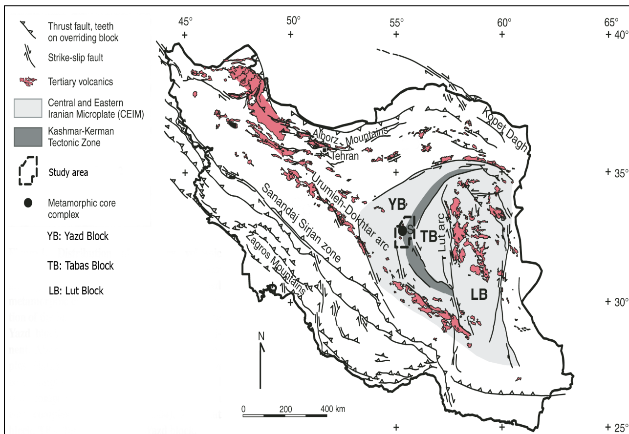
شکل ۱. موقعیت ناحیه ساغند بر روی پهنه زمین‌ساختی کرمان- کاشمر در خرده قاره ایران مرکزی (Verdel et al., 2007)
