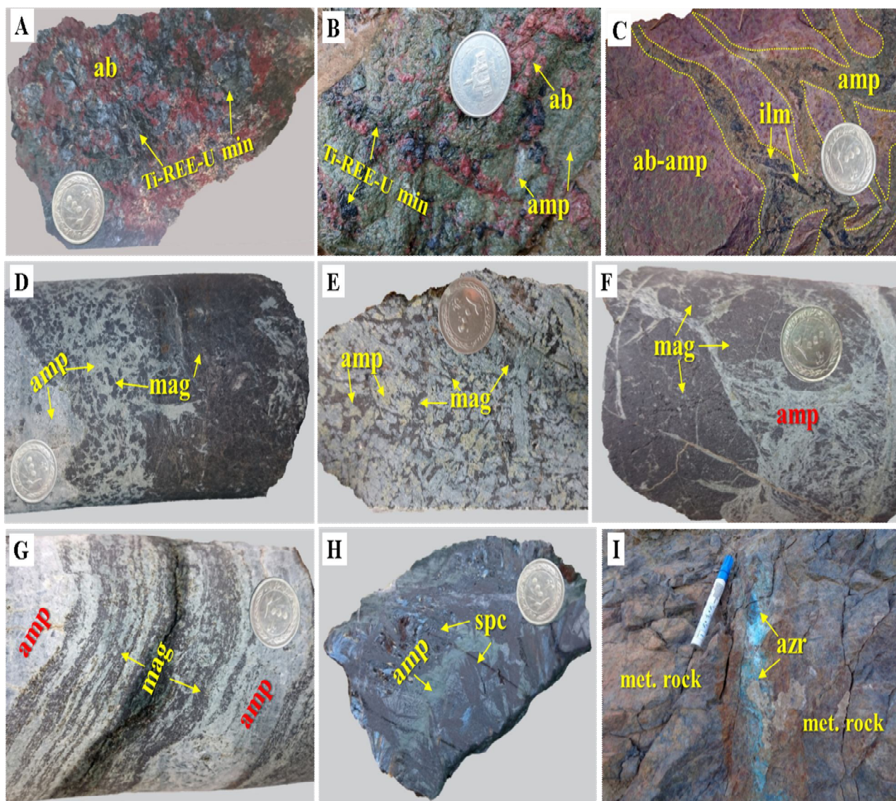
شکل ۶. A: نهشت کانه‌های Ti-REE-U در آلبیت‌های آنومالی پنج ساغند، B: کانی‌سازی افشان Ti-REE-U در دگرنهاد آمفیبولی - آلبیتی، C: رگه‌چه‌های آمفیبول حاوی ایلمنیت که آلبیت - آمفیبول‌های دگرنهادی را قطع کرده‌اند، D: نهشت مگنتیت توده‌ای و افشان در دگرنهاد آمفیبولی، E: مگنتیت فضای بین کانی‌های آمفیبول را پر کرده است، F: برشی شدن مگنتیت‌ها، G: نهشت نوارهای متناوب مگنتیت و آمفیبول، H: اسپکیولاریت‌های ورقه‌ای-رشته‌ای شکل در زمینه دگرنهاد آمفیبولی و I: دگرسانی سوپرژن رگه‌چه سولفیدی مس و تشکیل آزوریت در داخل سنگ دگرنهادی. تمام آمفیبول‌ها از گروه اکتینولیت - ترمولیت هستند. ab: آلبیت، amp: آمفیبول، ilm: ایلمنیت، mag: مگنتیت، spc: اسپکیولاریت، azr: آزوریت و met.rock: سنگ دگرنهادی، Ti-REE-U min: کانه‌های تیتانیوم، عناصر نادر خاکی و اورانیوم. علائم اختصاری کانی‌ها بر اساس ویتنی و اوانز (Whitney and Evans, 2010)
