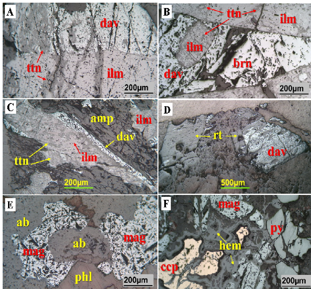
شکل ۷. A: ایلمنیت و دیویدایت و جانشینی آنها با تیتانیت در آنومالی پنج ساغند، B: دیویدایت و برانریت فضای بین بلورهای ایلمنیت را پر کرده و آن را در برگرفته‌اند و ایلمنیت هم به تیتانیت دگرسان شده است، C: نهشت دیویدایت در اطراف ایلمنیت و جانشینی ایلمنیت توسط تیتانیت، D: جانشینی دیویدایت توسط روتیل، E: رونهشت مگنتیت بر روی آل‌بیتیت و F: کانه‌زایی کالکوپیریت و پیریت در سنگ‌های دگرنهادی و جانشینی مگنتیت توسط هماتیت. ilm: ایلمنیت، dav: دیویدایت، ttn: تیتانیت، brn: برانریت، amp: آمفیبول، rt: روتیل، ab: آل‌بیت، mag: مگنتیت، phl: فلوگوپیت، ccp: کالکوپیریت، py: پیریت و hem: هماتیت. علائم اختصاری کانی‌ها بر اساس ویتنی و اوانز (Whitney and Evans, 2010)
