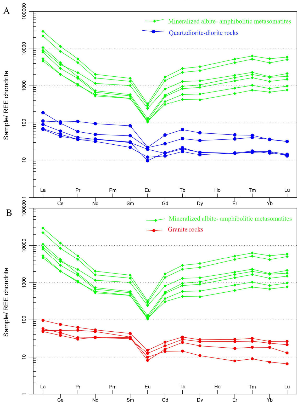
شکل ۱۱. الگوی نرمالیزه‌شده عناصر کمیاب خاکی (Nakamura, 1974) در دگرتهادی‌های آلبیتی- آمفیبولی کانه‌زایی‌شده کانسار ساغند و مقایسه آنها با A: کوارتزدیوریت- دیوریت مادر و B: گرانیت زیریگان (یا دوزخ دره)
