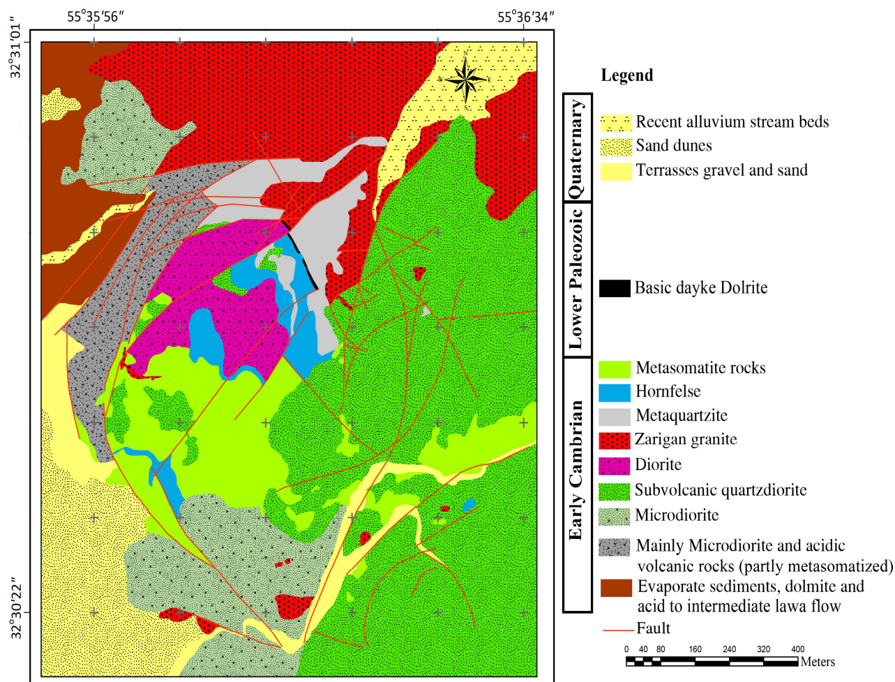
شکل ۳. نقشه زمین‌شناسی کانسار ساغند (Samani and Talezadeh lari, 1988)
