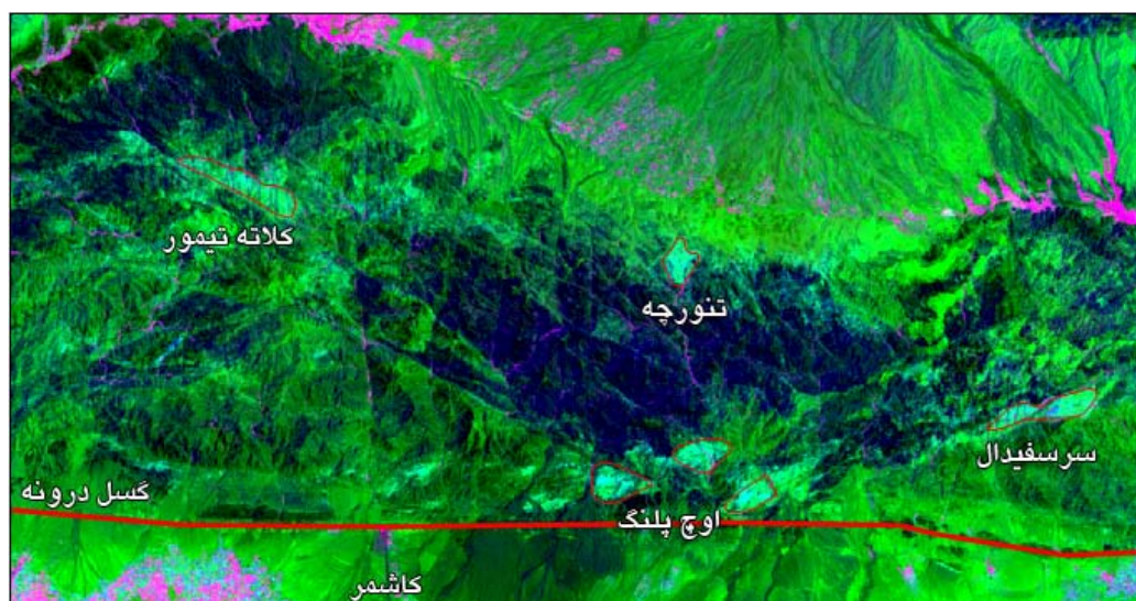
شکل ۳. در نسبت جدید (4/3) R و (5) G و (5/7) B مرز مناطق دگرسانی شمال گسل درونه قابل تمیز از واحدهای دیگر هستند.
