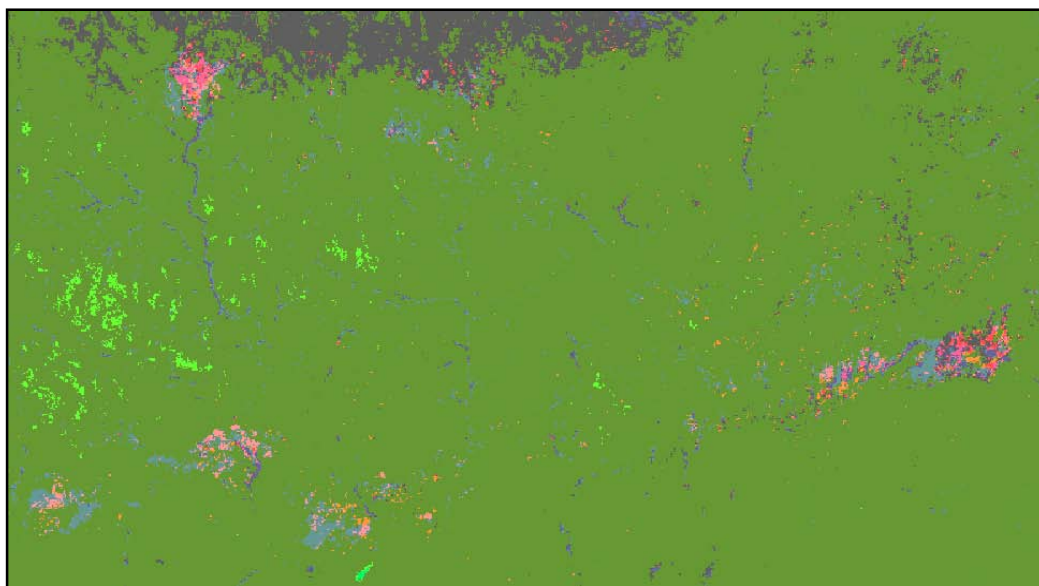
شکل ۴. در نسبت جدید (5/2) R و (1/4) G و (5/7) B مناطق دگرسانی با رنگهای صورتی، آبی، ارغوانی، نخودی دیده می‌شود.
