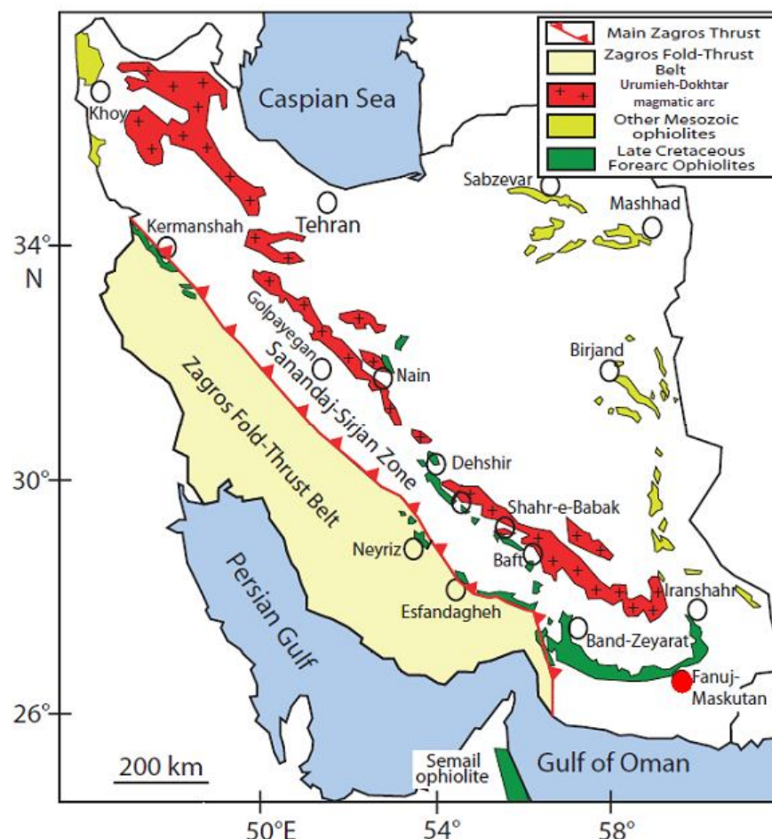
شکل 1. نقشه پراکندگی افیولیت‌های ایران و موقعیت جغرافیایی پیکره افیولیتی فنوج - مسکوتان (رمشک) در جنوب‌شرقی آن که با دایره قرمز توپر مشخص شده است (با تغییرات از (Shafaii Moghadam and Stern, 2011)).
