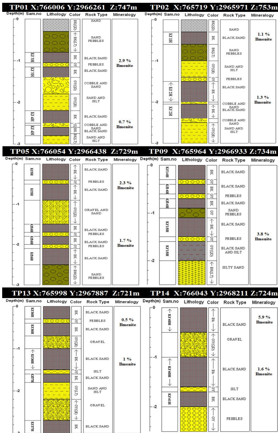
شکل 7. برشهای عمودی 6 چاهک منتخب از ناحیه دره جوگز بالا در منطقه فنوج که در آن موقعیت (افقهای خاکستری رنگ) و عیار افقهای تیتانیوم‌دار مشخص شده است. موقعیت جغرافیایی چاهکها بر روی شکل 3 نمایش داده شده است. شماره هر چاهک در بالای برش درج شده است.
