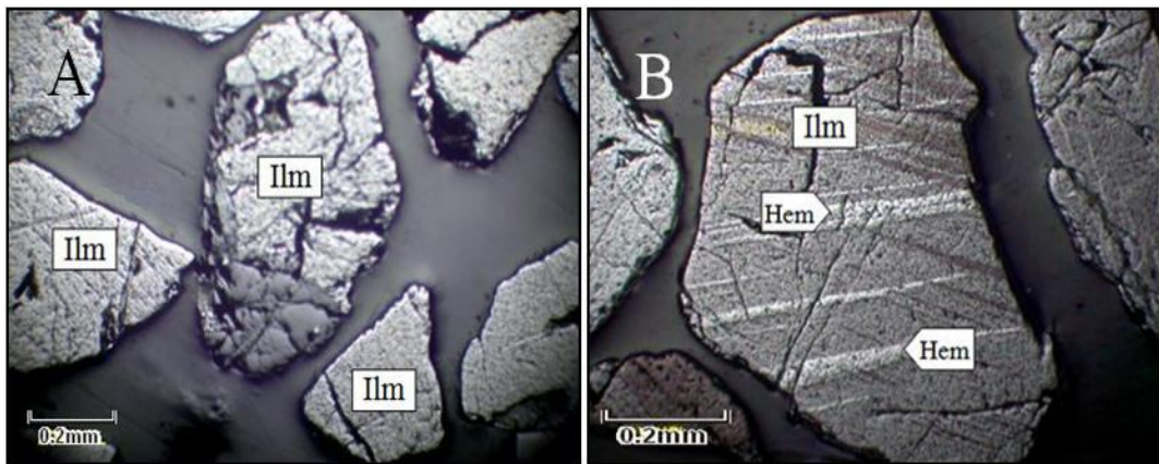
شکل 8. تصاویر میکروسکوپی دانه‌های کانه ایلمنیت (Ilm) در بخش سنگین رسوبات تیتانیوم‌دار ناحیه دره جوگز بالا در منطقه فنوج. A: بلورهای زاویه‌دار تا نیمه گرد شده کانه ایلمنیت در بخش سنگین و B: تشکیل تیغه‌های ناآمیختگی هماتیت (Hem) در کانه ایلمنیت (نور پلاریزه انعکاسی ساده).
