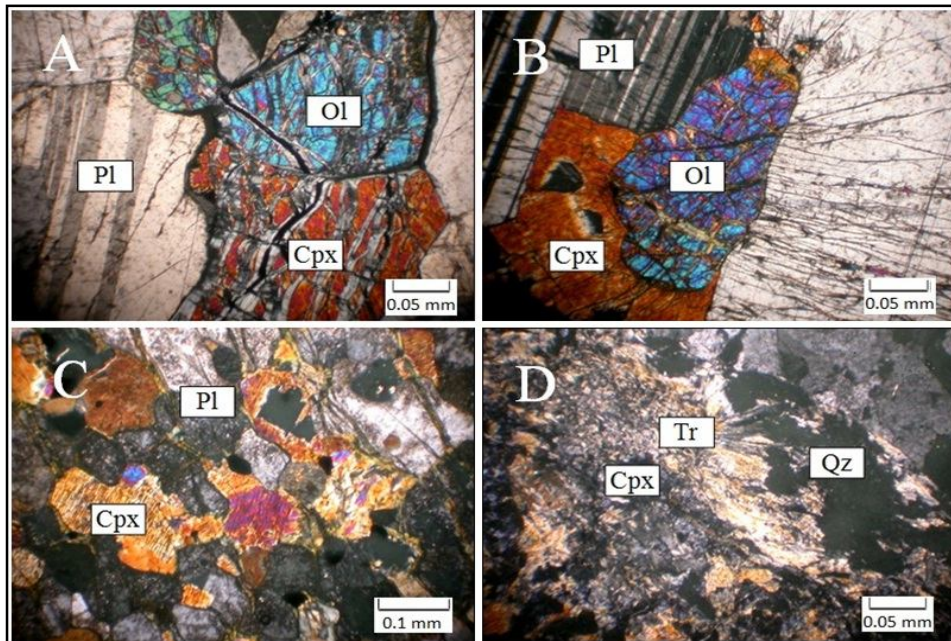
شکل 4. A: بافت انباشتی در گابروهای لایه‌ای منطقه فنوج، B: بلورهای زینومورف پلاژیوکلاز (Pl)، کلینوپیروکسن (Cpx) و الیون (Ol) در واحد الیون گابروی منطقه فنوج، C: بلورهای زینومورف کلینوپیروکسن و پلاژیوکلازهای رسی و سریسیتی شده در گابروهای لایه‌ای منطقه فنوج و D: کلینوپیروکسن ترمولیتی شده (Tr) و رگچه کوارتزی (Qz) در واحد گابروی منطقه فنوج (همه تصاویر در نور عبوری پلاریزه متقاطع تهیه شده‌اند).
