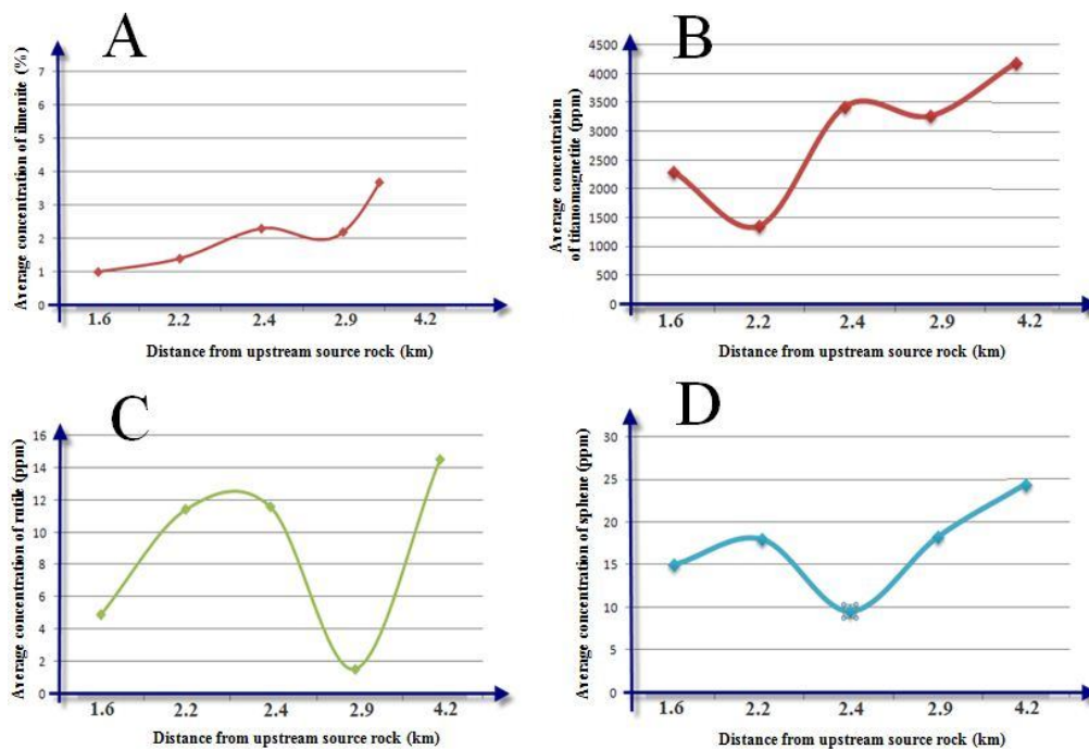
شکل 9. روند غنی‌شدگی کانیهای تیتانیوم‌دار در بستر رودخانه دره جوگز بالا در مقابل فاصله از سنگ مادر واقع در بالا دست رودخانه. A: کانی ایلمنیت، B: کانی تیتانومگنتیت، C: کانی روتیل و D: کانی اسفن.
