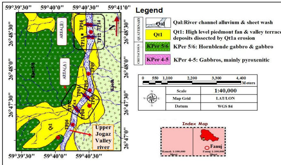
شکل 3. موقعیت محدوده‌های A و B و چاهک‌های حفر شده در بستر رودخانه دره جوگز بالا در منطقه فنوج. واحد kper5/6 اولیون گابرو و هورنبلند گابرو، و واحد kpedb دولریت (دیابازهای دگرسان شده) است.
