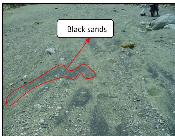
شکل 10. لایه‌های سطحی ماسه‌ای سیاه رنگ نازک سرشار از کانی سنگین (ایلمنیت) در بستر رودخانه دره جوگز بالا که احتمالاً بر اثر عملکرد فرآیند برداشتن و حمل کردن هیدرولیکی تشکیل شده‌اند.
