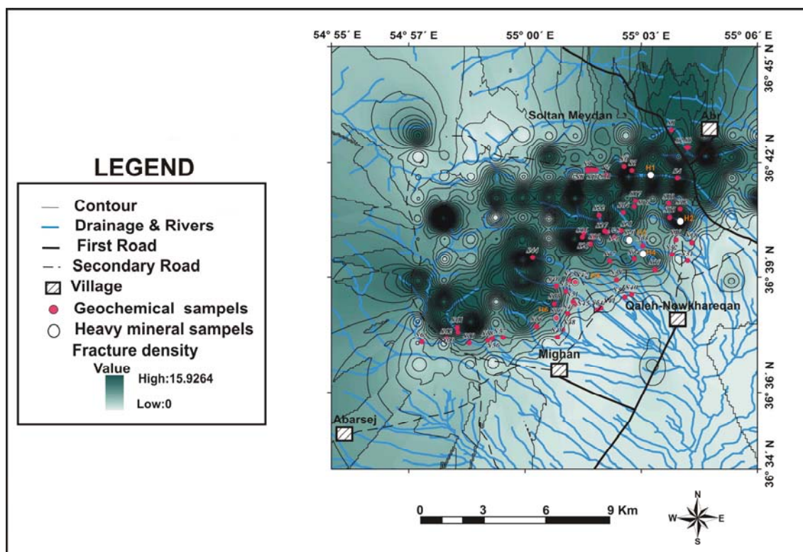
شکل ۷. نقشه هم‌تراز ضرب خط‌وارگی در منطقه مورد مطالعه و انطباق محدوده‌های واجد ناهنجاریهای زمین‌شیمیایی شناسایی شده بر مناطق با چگالی بالای شکستگی.
