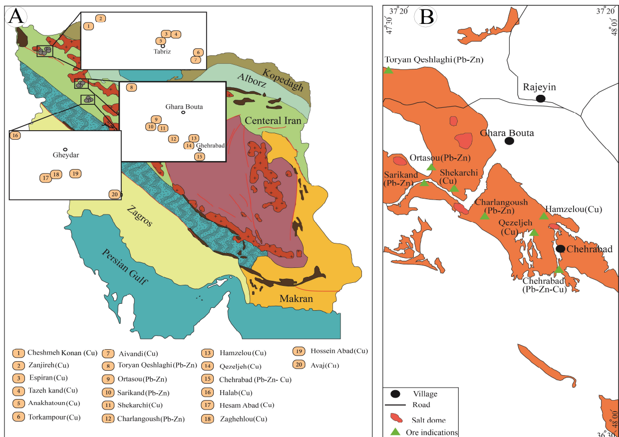
شکل ۱. A: موقعیت کانسارها و نشانه‌های مس و سرب-روی با میزان رسوبی در بخش شمال‌باختری پهنه ایران مرکزی با تغییرات از علوی (Alavi, 1991). نوع ماده معدنی در داخل پرانتز مشخص شده است و B: گسترش سازند قرمز بالایی در منطقه ماه‌نشان و موقعیت کان‌زایی‌های مس و سرب-روی با میزان رسوبی با تغییرات از لطفی (Lotfi, 2001) و خدابنده و همکاران (Khodabandeh et al., 1998). به ارتباط نزدیک گنبد‌های نمکی و کان‌زایی‌های مزبور در این سازند توجه‌شود.
