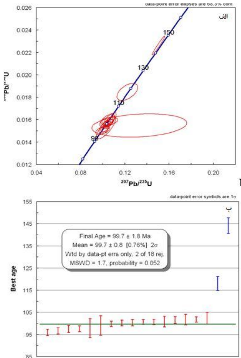
شکل 14. الف) پلات کنکردیا و ب) تعیین سن میانگین.
