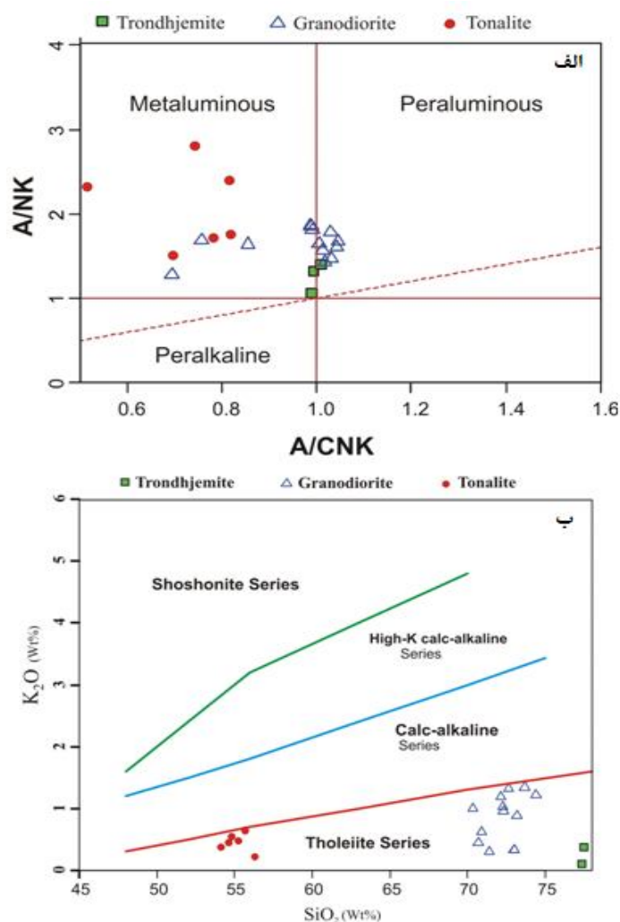
شکل 7. نمونه‌های مورد بررسی منطقه هلاک‌آباد الف) در نمودار A/NK در مقابل A/CNK [12] در محدوده متآلومین تا پراآلومین و ب) در نمودار SiO 2 در مقابل K 2 O [13] در محدوده تولییتی قرار دارند.
