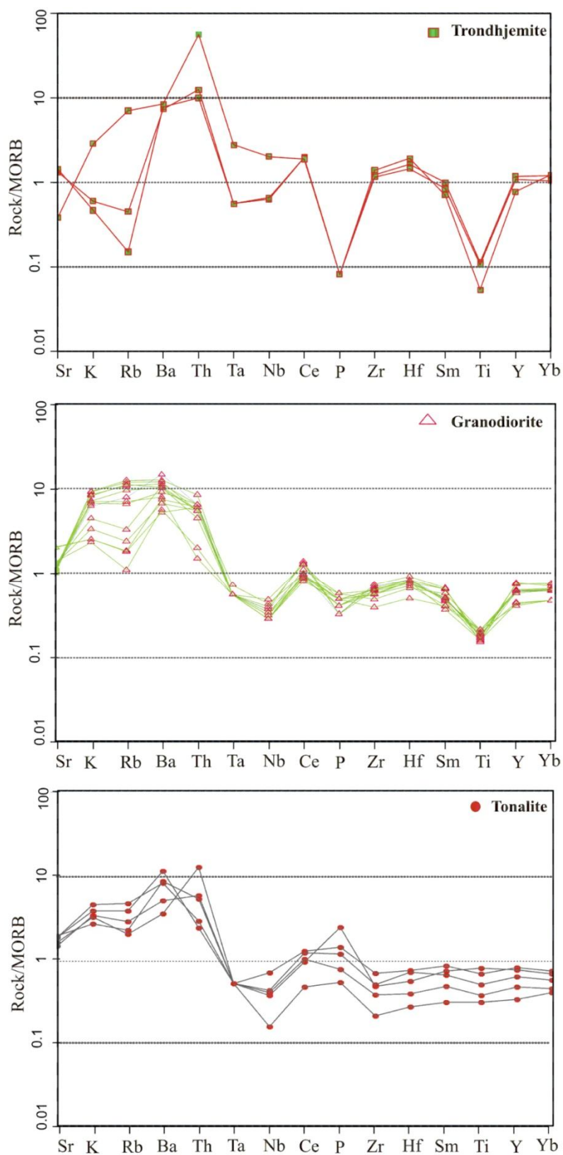
شکل 13. موقعیت نمونه‌های منطقه هلاک‌آباد در نمودارهای عنکبوتی عناصر فرعی و کمیاب که نسبت به مقادیر مورب [18] نرمال شده‌اند.
