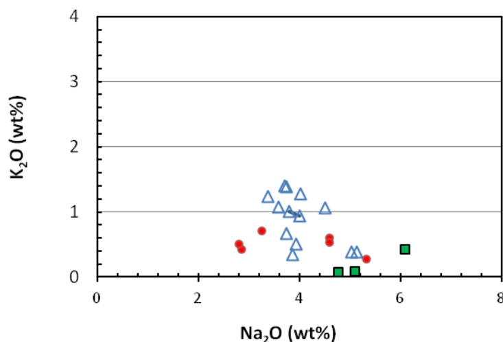
شکل 8. مقایسه محتوای Na 2 O در مقابل K 2 O. نمونه‌های منطقه هلاک‌آباد غنی از سدیم هستند (راهنما مشابه شکل‌های قبلی).
