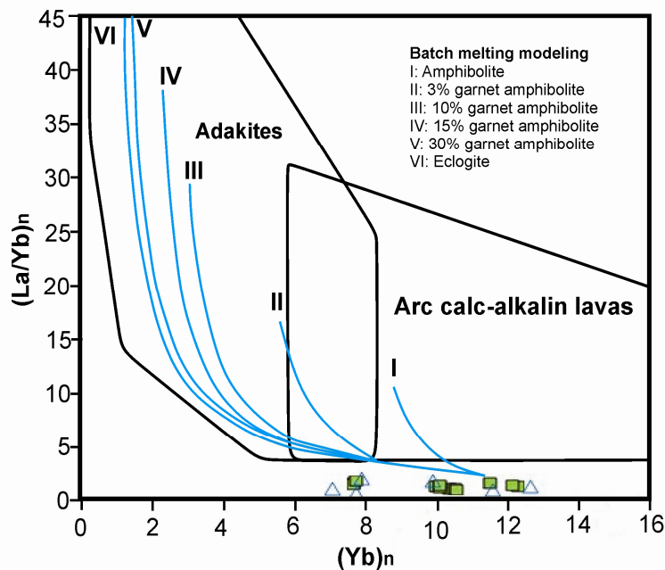
شکل 18. نمودارهای (\text{Yb})_N در مقابل (\text{La}/\text{Yb})_N [36] منشأ ماگما را از خارج محدوده پایداری گارنت نشان می‌دهد.
