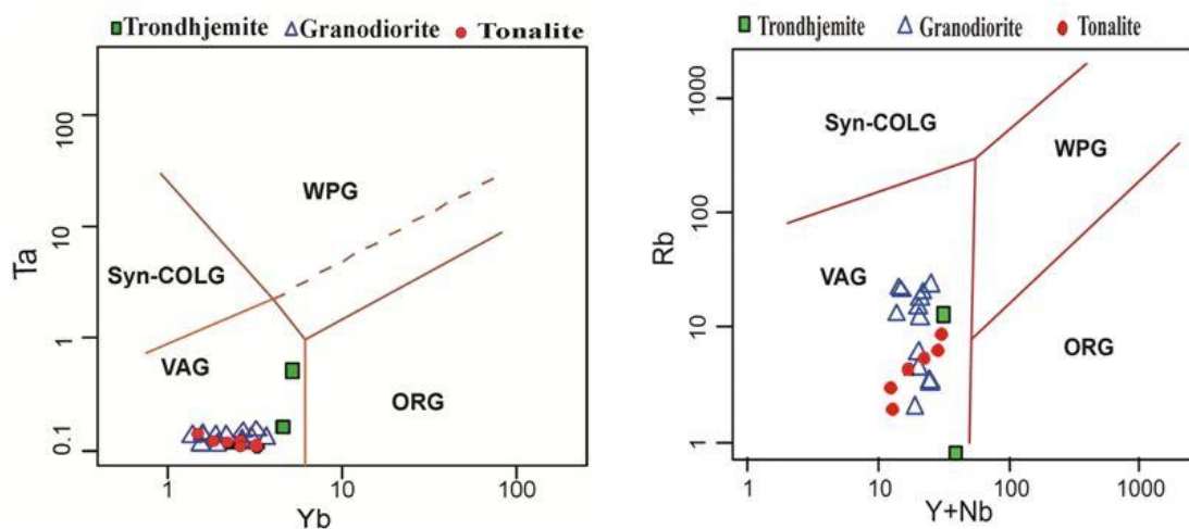
شکل 11. نمونه‌های مورد بررسی منطقه هلاک‌آباد در نمودار تعیین موقعیت تکتونیکی گرانیتوئیدها [16]، در کمربندهای آتشفشانی زون فرورانش قرار می‌گیرند.
