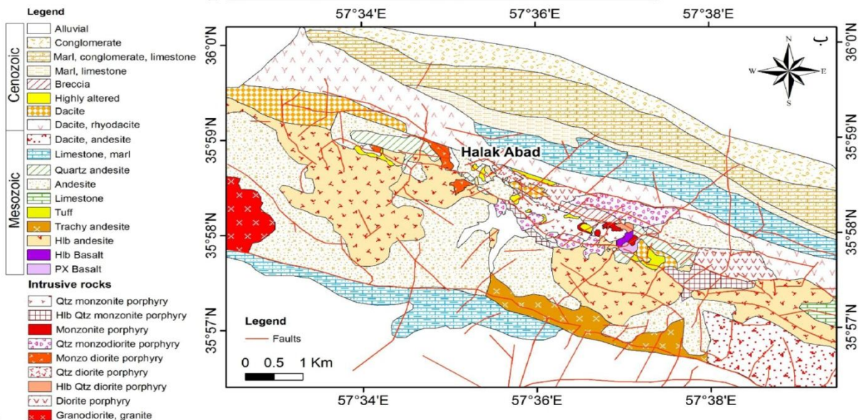
شکل 1. الف) زونهای ساختاری ایران (با تغییرات پس از [9]). موقعیت منطقه هلاک‌آباد با کادر مشخص شده است. ب) نقشه زمین‌شناسی محدوده هلاک‌آباد.
