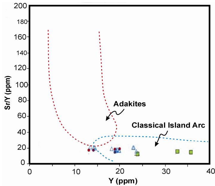
شکل 17. نمونه‌های منطقه هلاک‌آباد در نمودار Y در مقابل Sr/Y [35] در محدوده جزایر قوسی قرار می‌گیرند.
