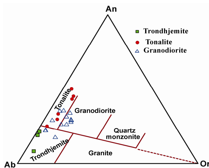
شکل 6. نمونه های مورد بررسی منطقه هلاک آباد در نمودار سه تایی آل بیت - آنورتیت - ارتوکلاز [11] در محدوده ترانجمیت، تونالیت و گرانودیوریت قرار می گیرند.
