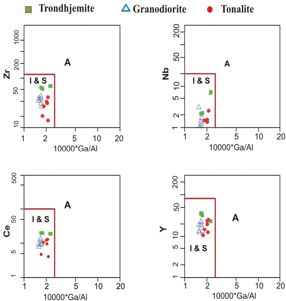
شکل 10. موقعیت نمونه‌های مورد بررسی منطقه هلاک‌آباد در نمودار [15] در محدوده متعلق به ماگماتیسزم سری I و S قرار گرفته است.
