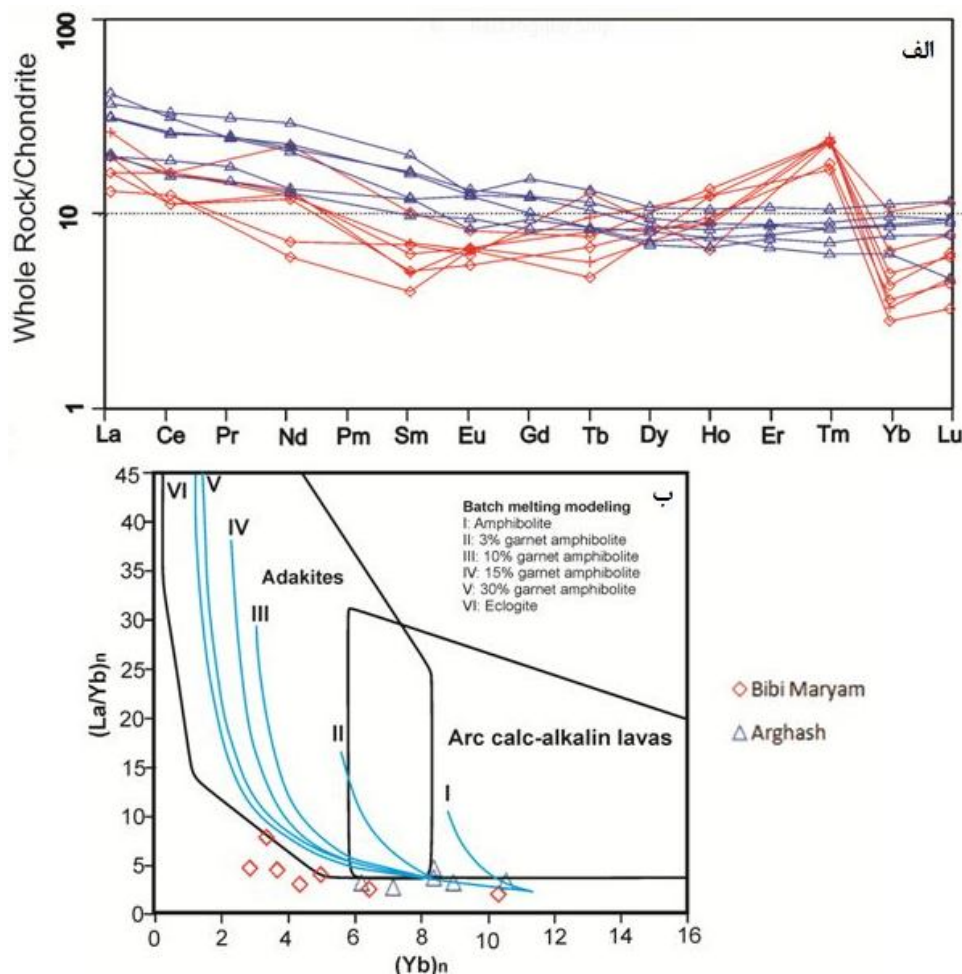
شکل 16. مقایسه توده هورنبلند گرانودیوریت ارغش و تونالیت-گرانودیوریت بی‌بی مریم در الف) نمودار عنکبوتی که نسبت به مقادیر کندریت [17] نرمالیزه شده‌اند ب) نمودار (\text{Yb})_N در مقابل (\text{La}/\text{Yb})_N [35].
