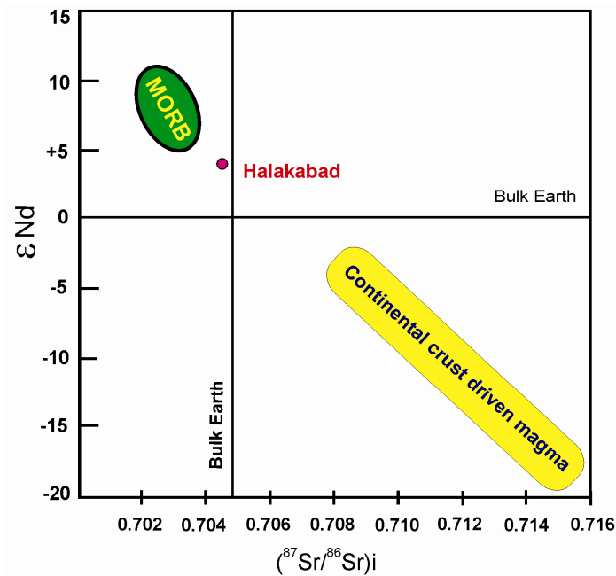
شکل 15. مقایسه میزان (^{87}\text{Sr}/^{86}\text{Sr})_i و \epsilon\text{Nd} نمونه مطالعاتی منطقه هلاک‌آباد
