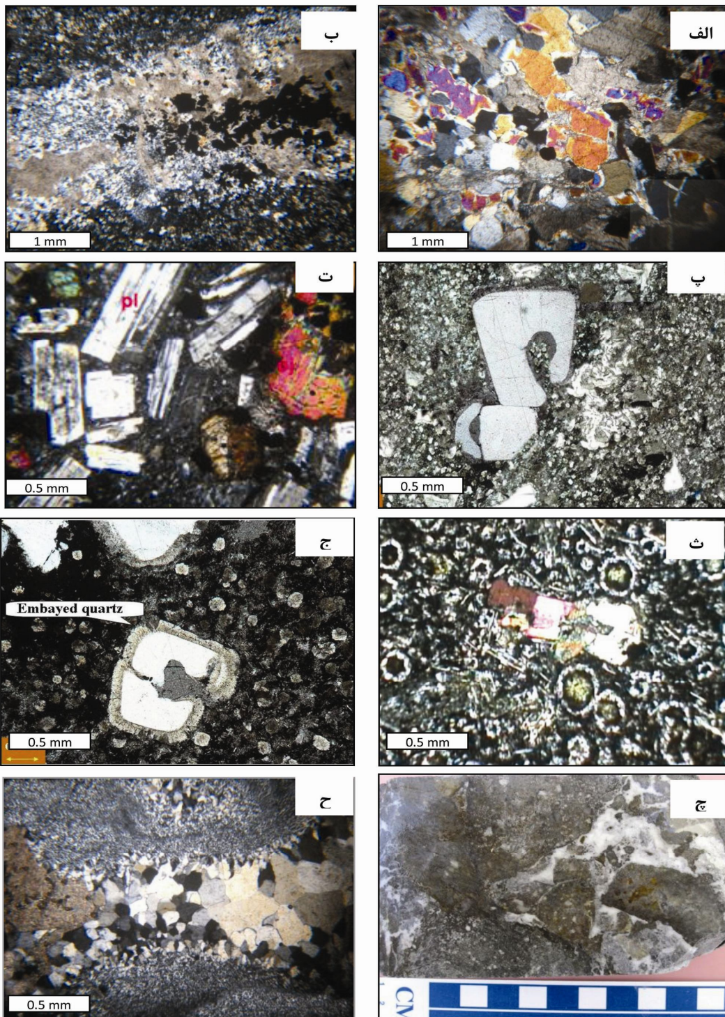
شکل 2. الف) دگرسانی آرژلیک پیشرفته (آلونیت، کوارتز و کربنات). ب) دگرسانی آرژلیک - سیلیسی - کربنات در کوارتز مونزونیت پورفیری. سیلیس و کانیه‌های رسی در حاشیه رگه‌چه و کربنات و اپک در وسط دیده می‌شود. پ) فنوکریست کوارتز خلیجی در زمینه یک سنگ داسیتی. ت) پیروکسن اندزیت. ث) بافت بادامکی در بازالتها ج) کوارتز نبود تعادل با حاشیه واکنشی در سنگ داسیتی همراه با دگرسانی سیلیسی چ) نمونه دستی از برش هیدروترومال. ح) رگه‌چه از حاشیه به داخل توسط کوارتزهای ریزبلور و سپس کوارتز درشت‌بلور و کربنات پر شده است. (تصاویر میکروسکوپی در نور XPL).
