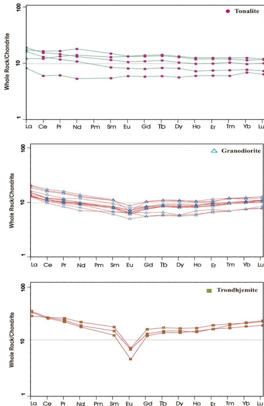
شکل 12. موقعیت نمونه‌های منطقه هلاک‌آباد در نمودارهای عنکبوتی عناصر فرعی و کمیاب که نسبت به مقادیر کندریت [17] نرمال شده‌اند.
