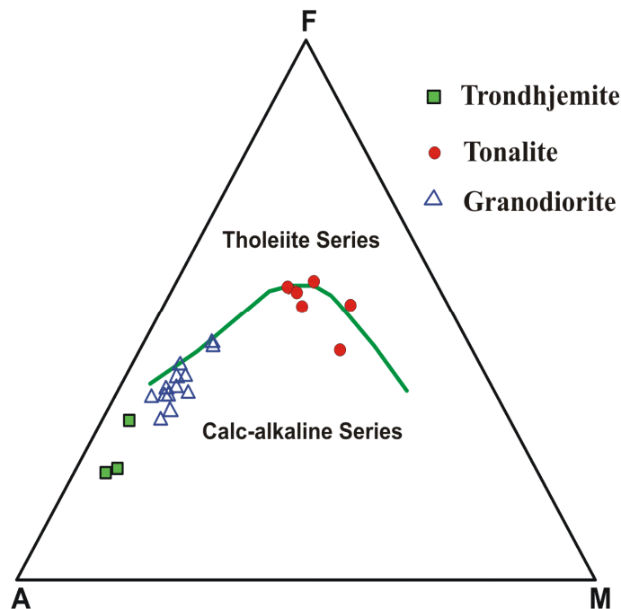
شکل 9. نمونه‌های مورد بررسی منطقه هلاک‌آباد در نمودار AFM [14] در محدوده تولییتی تا کالک‌آلکان قرار دارند.
