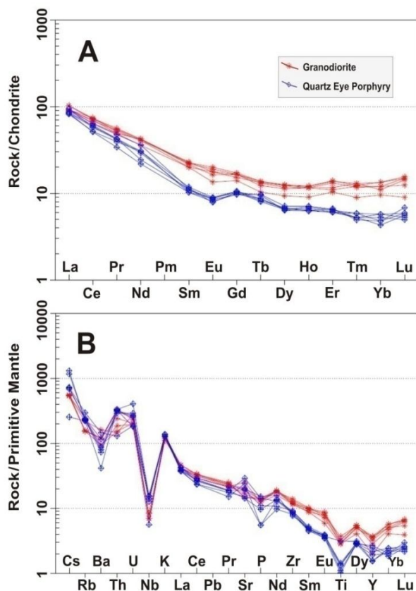
شکل 7. A: الگوی تغییرات عناصر نادر خاکی توده‌های نفوذی گرانودیوریتی و کوارتز چشمی پورفیبری کانسار مس پورفیبری سرچشمه که نسبت به کندریت بهنجار شده‌اند (Boynton, 1984) و B: الگوی تغییرات عناصر کمیاب و نادر خاکی توده‌های نفوذی گرانودیوریتی و کوارتز چشمی پورفیبری در کانسار مس پورفیبری سرچشمه که نسبت به گوشته اولیه بهنجار شده‌اند (Sun and McDonough, 1989).
