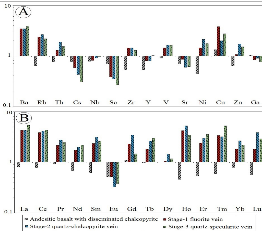
شکل ۱۳. A: نمودار عناصر کمیاب برای بخشهای کانهدار در رخداد معدنی مس آق کند که نسبت به گدازه بازالت آندزیتی سالم و بدون کان‌زایی ائوسن (نمونه AQ-14، جدول ۱) به‌هنگار شده‌اند و B: نمودار عناصر نادر خاکی برای بخشهای کانهدار در رخداد معدنی مس آق کند که نسبت به گدازه بازالت آندزیتی سالم و بدون کان‌زایی ائوسن (نمونه AQ-14، جدول ۱) به‌هنگار شده‌اند.
