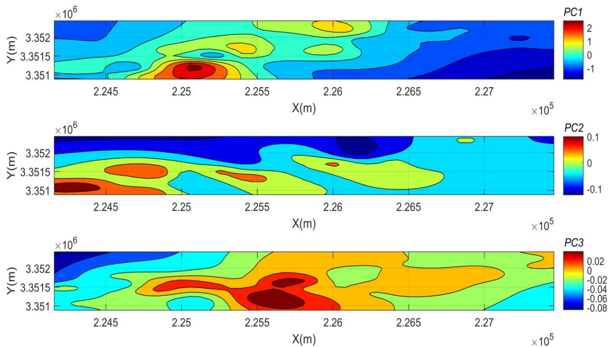
شکل 13. نقشه دو بعدی X-Y (طول و عرض جغرافیایی) توزیع بار فاکتوری مؤلفه‌های اول تا سوم ( PC_1 - PC_3 ) در محدوده شرقی مروست
