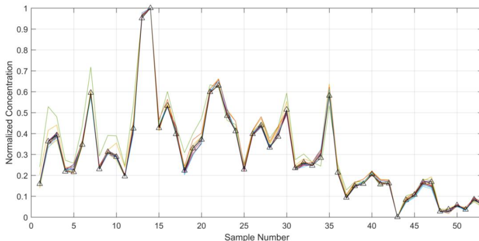
شکل 2. نمودار تغییر پذیری غلظت عناصر نادر خاکی (استاندارد شده در بازه 0-1) برای نمونه های مورد بررسی در محدوده خاوری مروت
