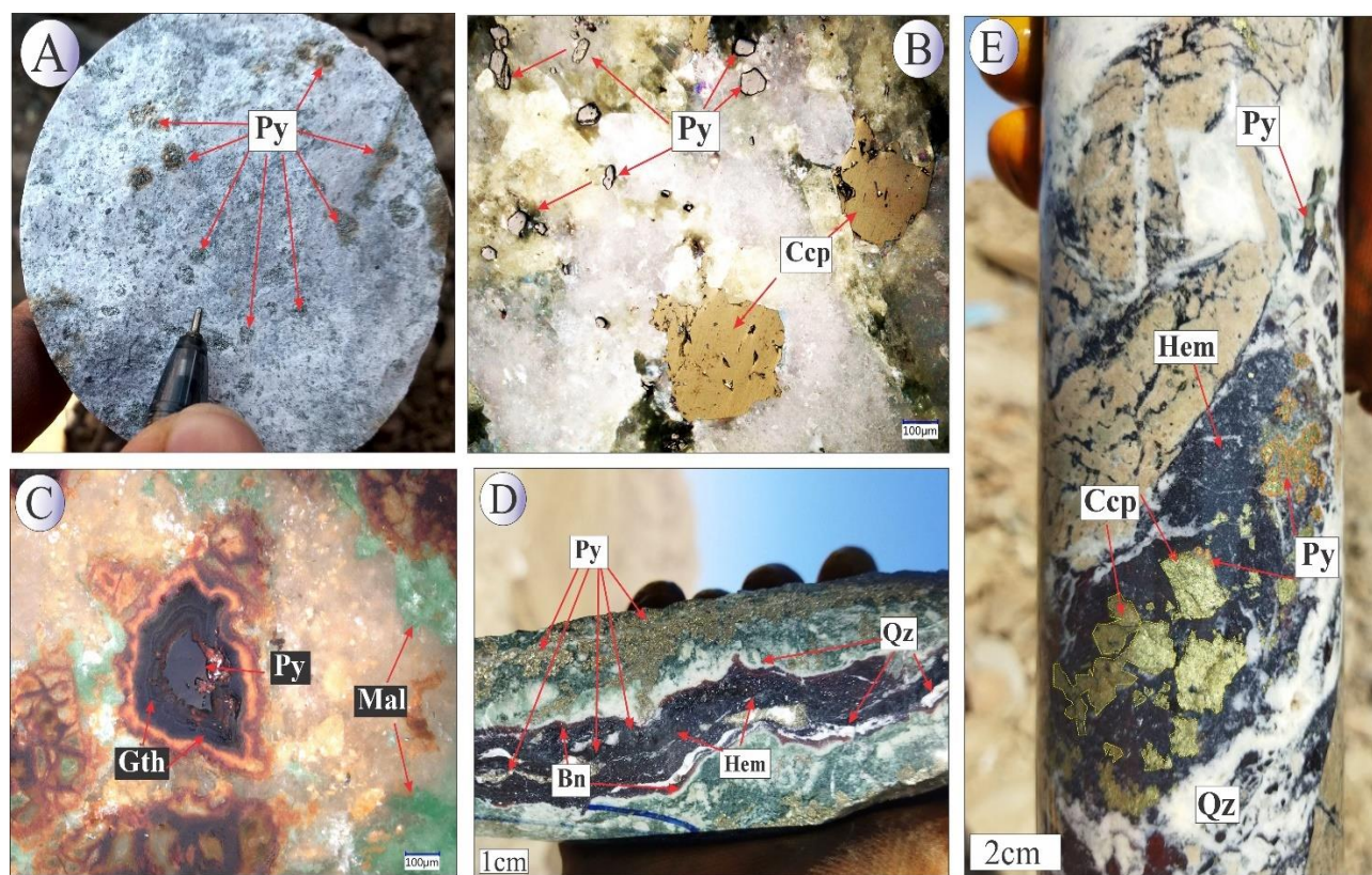
شکل ۳. تصویرهایی از کانی‌سازی پیریت در منطقه مأمونیه: A: کانی‌سازی پراکنده پیریت در زمینه واحد ریوداسیت، B: بلورهای پیریت افشان در زمینه رگه سیلیسی، C: کانی‌سازی پراکنده پیریت که تحت تأثیر هوازدگی در حاشیه‌ها به گوتیت تبدیل شده است، D: کانی‌سازی هماتیت اسپیکولار و بورنیت به صورت کلوفرم و قشری در مغزه حفاری و E: کانی‌سازی برشی کالکوپیریت + پیریت + هماتیت اسپیکولار در رگه سیلیسی. نام اختصاری کانی‌ها از ویتنی و اوانز (Whitney and Evans, 2010) اقتباس شده است (Hem: هماتیت، Ccp: کالکوپیریت، Py: پیریت، Qz: کوارتز، Bn: بورنیت، Gth: گوتیت، Mal: مالاکیت).
