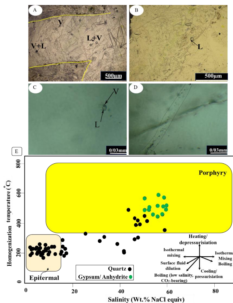
شکل ۸. A-D: تصویرهای میکروسکوپی از انواع میان‌بارهای سیال بررسی شده در کانی‌های کوارتز، ژپس و انیدریت. A: میان‌بارهای دوفازی غنی از مایع (L+V) و غنی از گاز (V+L) در رگه ژپس، B: میان‌بارهای تک‌فازی مایع (L) در رگه انیدریت، C: میان‌بار دوفازی غنی از مایع به صورت انفرادی و اولیه در کانی کوارتز، D: میان‌بارهای سیال ثانویه در زمینه کوارتز، E: نمودار دمای همگن‌سازی در مقابل شوری میان‌بارهای سیال در کانسار دوگان
