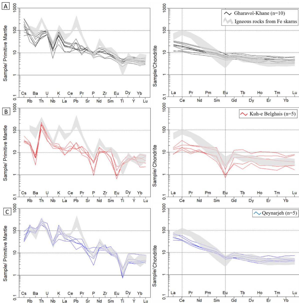
شکل ۵. نمودارهای عنکبوتی عناصر کمیاب بهنجار شده با گوشته اولیه (Sun and McDonough, 1989) و عناصر کمیاب خاکی بهنجار شده با کندریت (Boynton, 1984) در دنباله‌های نفوذی ناحیه قینرجه-انگوران. A: توده کوارتز دیوریت قراول‌خلنه، B: واحد گرانیت پورفیری کوه بلقیس و C: واحد گرانودیوریت قینرجه. ترکیب توده‌های نفوذی مرتبط با ذخایر اسکارن آهن دنیا توسط ماینرت (Meinert, 1995) برای مقایسه نشان داده شده است.
