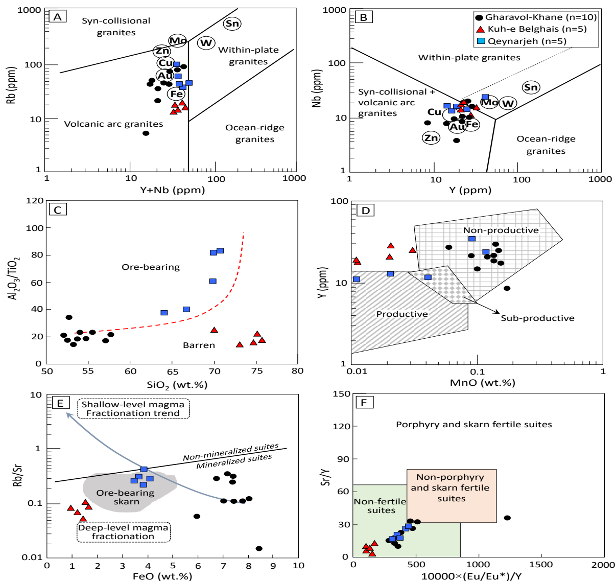
شکل ۹. نمودارهای تحولات زمین شیمیایی و ارزیابی پتانسیل فلزایی در دنباله‌های نفوذی ناحیه قینرجه-انگوران. A: نمودار دوتایی Rb در مقابل Y+Nb (Pearce) (Pearce et al., 1984) B: نمودار دوتایی Nb در مقابل Y (Pearce et al., 1984) C: نمودار دوتایی نسبت Al_2O_3/TiO_2 در مقابل SiO_2 (Liu and Peng, 2003) D: تعیین مولد تا غیرمولد بودن دنباله‌های نفوذی منطقه در نمودار دوتایی Y در مقابل MnO (Baldwin and Pearce, 1982) E: نمودار دوتایی Rb/Sr در مقابل FeO (Blevin and Chappell, 1992) F: بررسی شاخص زمین شیمی سنگ کل برای تعیین باروری یا عقیم بودن دنباله‌های نفوذی توسط نمودار دوتایی Sr/Y در مقابل 10000 \times (Eu/Eu^*)/Y (Svetlitskaya and Nevolko, 2022)
