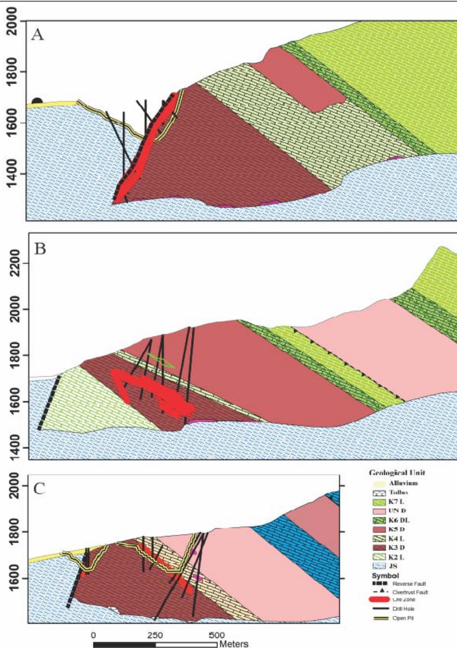
شکل ۳. مقاطع زمین‌شناسی و موقعیت ذخایر ایرانکوه شمالی. A: مقطع AB و نمایش موقعیت ذخیره گوشفیل، B: مقطع CD و نمایش موقعیت ذخیره زون ۵ رومرم و C: مقطع EF و نمایش موقعیت ذخیره مدفون و تپه‌سرخ
