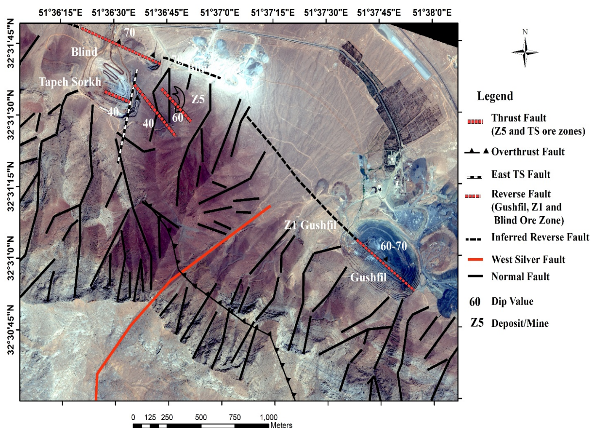
شکل ۴. نمایش خطواره‌ها و ساخت‌های زمین‌ساختی مرتبط با کانی‌سازی و جوان‌تر از آن در قلمرو ایرانکوه شمالی
