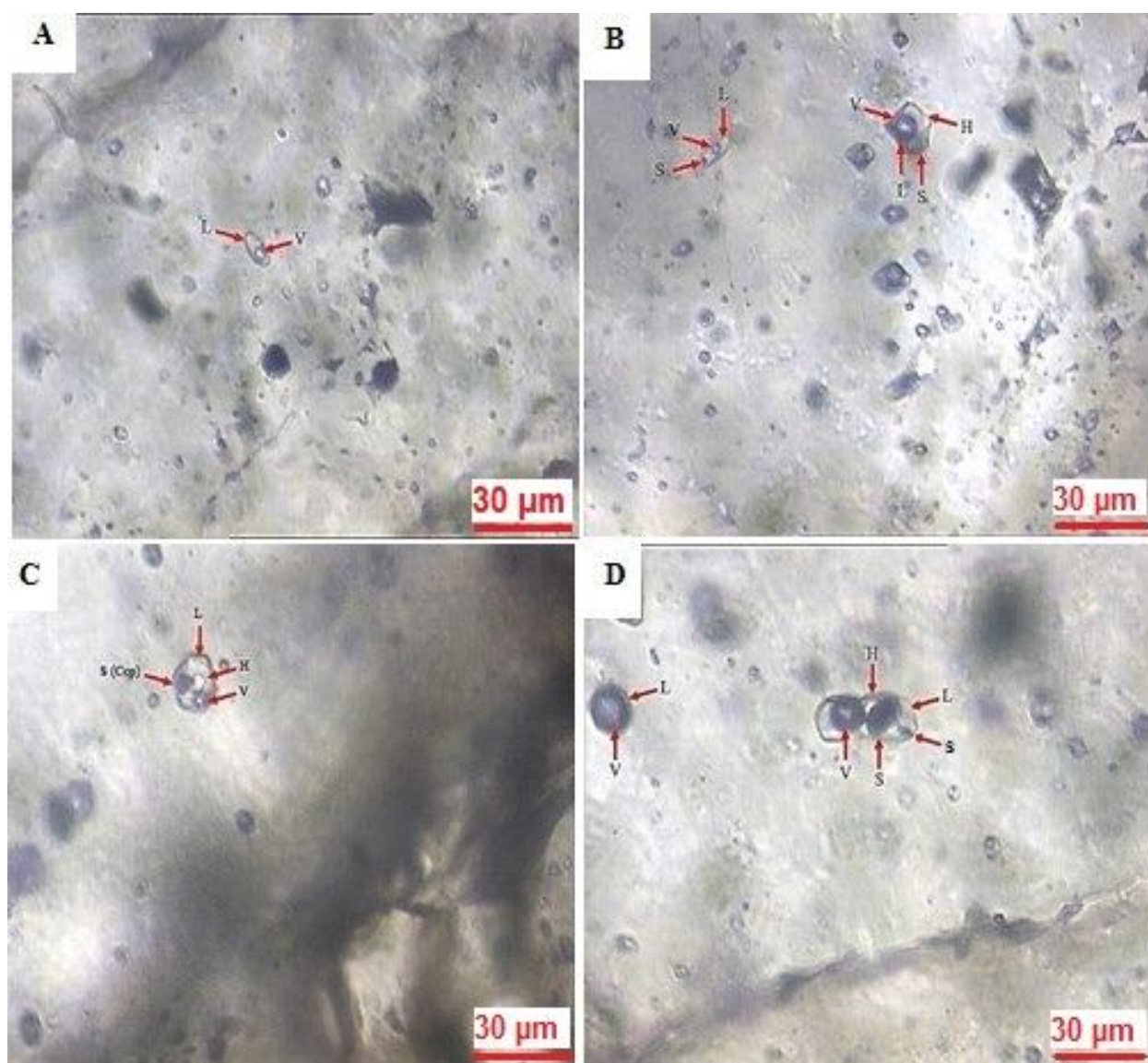
شکل ۸. تصاویر نور عبوری سیالات مختلف سیستم‌های مس پورفیری (A و B) و کیکال (C و D). A و B: بعضی از انواع سیالات معدن سونگون انواع LV (A) و LVS و LVHS (B)، C و D: دو سیال درگیر از نوع LVHS اندیس کیکال، بخار (V)، مایع (L)، هالیت (H)، جامد (S). کالکوپریت (Ccp)
