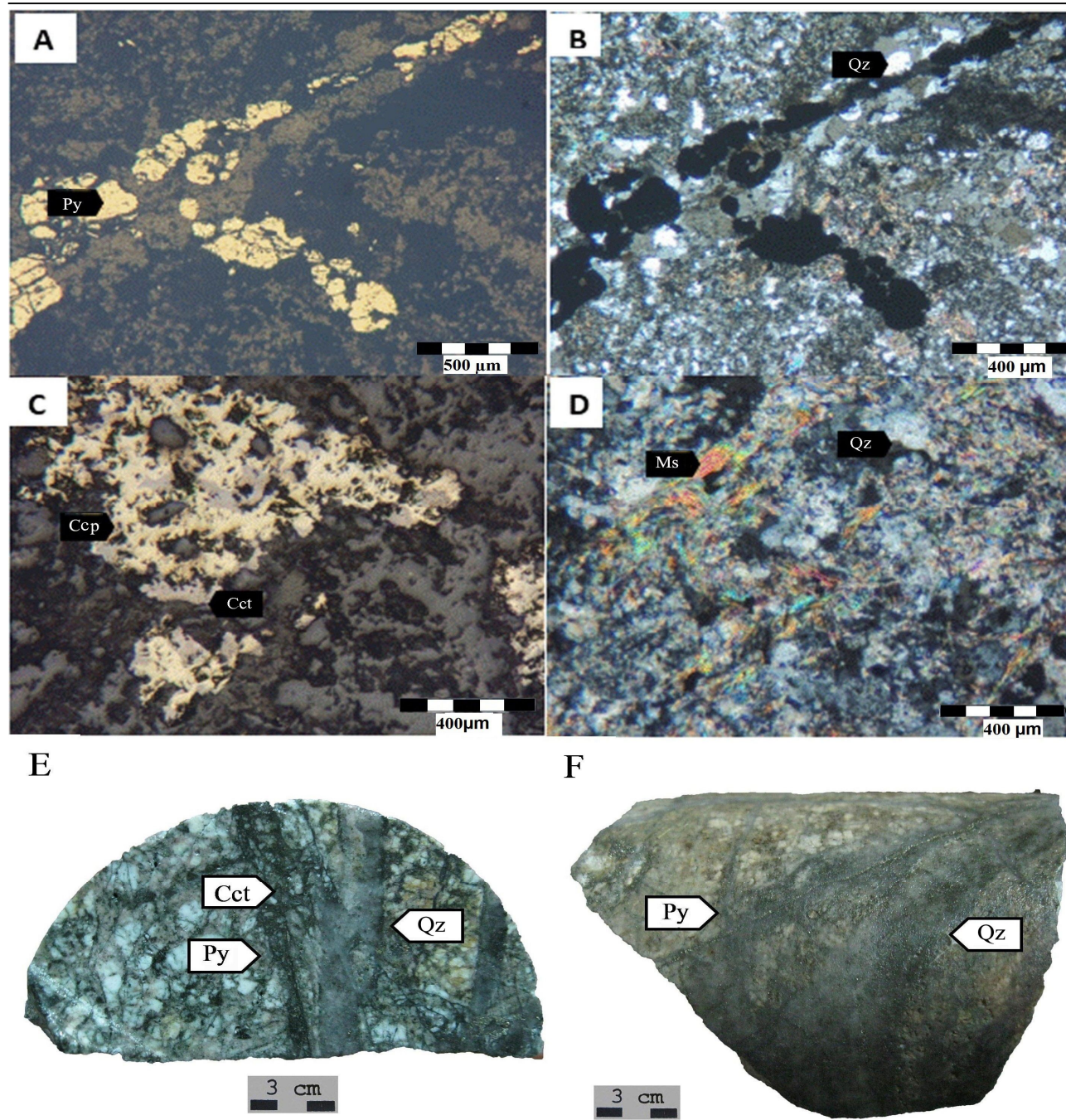
شکل ۷. A و B: وجود پیریت در رگه کوارتزی (نوع A)، C: کالکوسیت و کالکوپیریت در رگه‌چه‌های کوارتزی (رگه B)، D: دگرسانی سریسیتی و تشکیل مسکویت در دگرسانی فیلیک، E: نمونه دستی از رگه‌چه نوع A دارای کوارتز، پیریت و کالکوسیت و کوارتز و F: رگه‌چه نوع B دارای پیریت و کوارتز، اندیس کیقال. (Py: پیریت، Cct: کالکوسیت، Ccp: کالکوپیریت، Ms: مسکویت، Qz: کوارتز). مخفف‌های کانی‌ها از ویتنی و اوآنز (Whitney and Evans, 2010)
