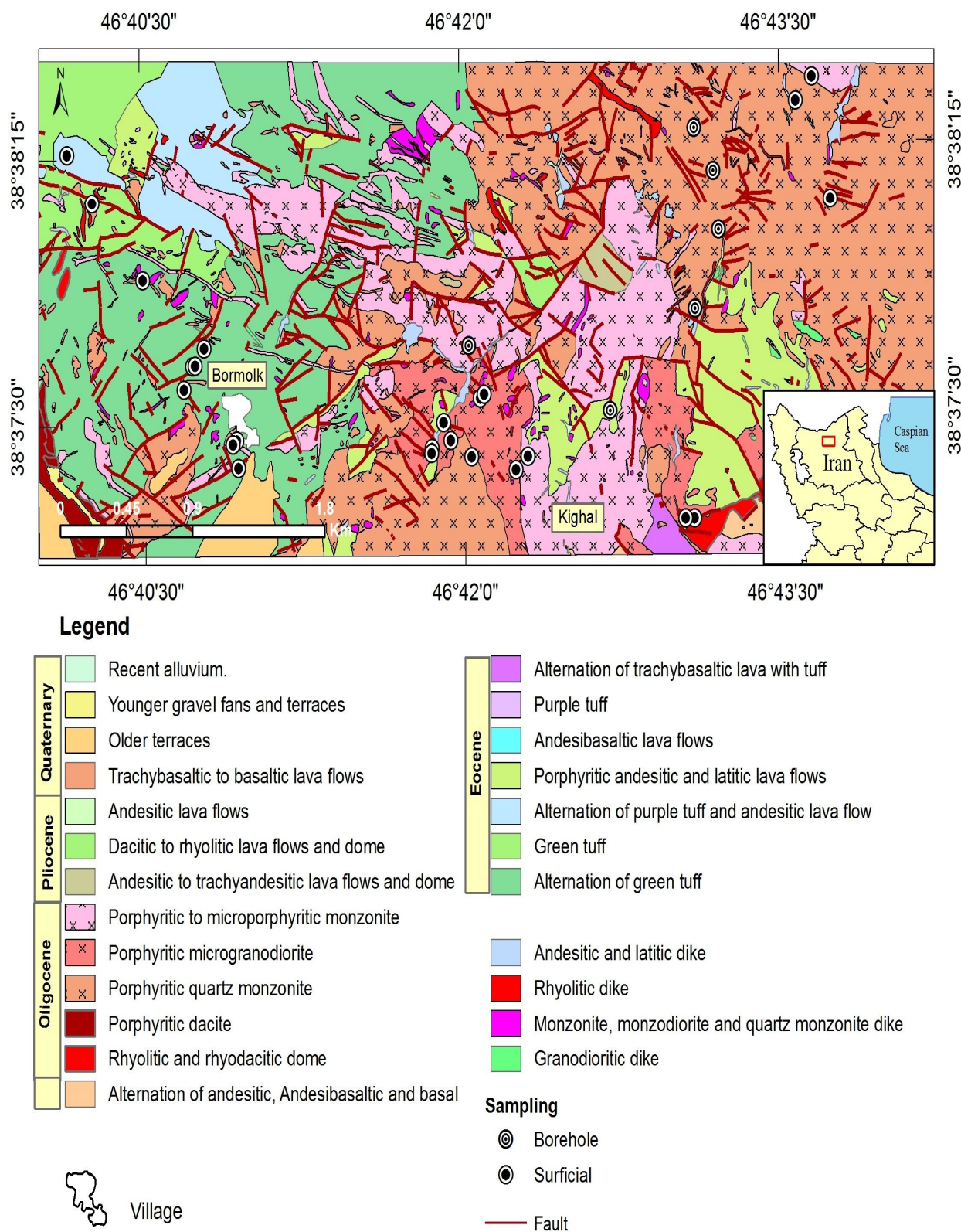
شکل ۳. نقشه زمین‌شناسی منطقه‌ای و نقاط نمونه‌برداری اندیس کیکال - بورملک (NICICO, 2006)
