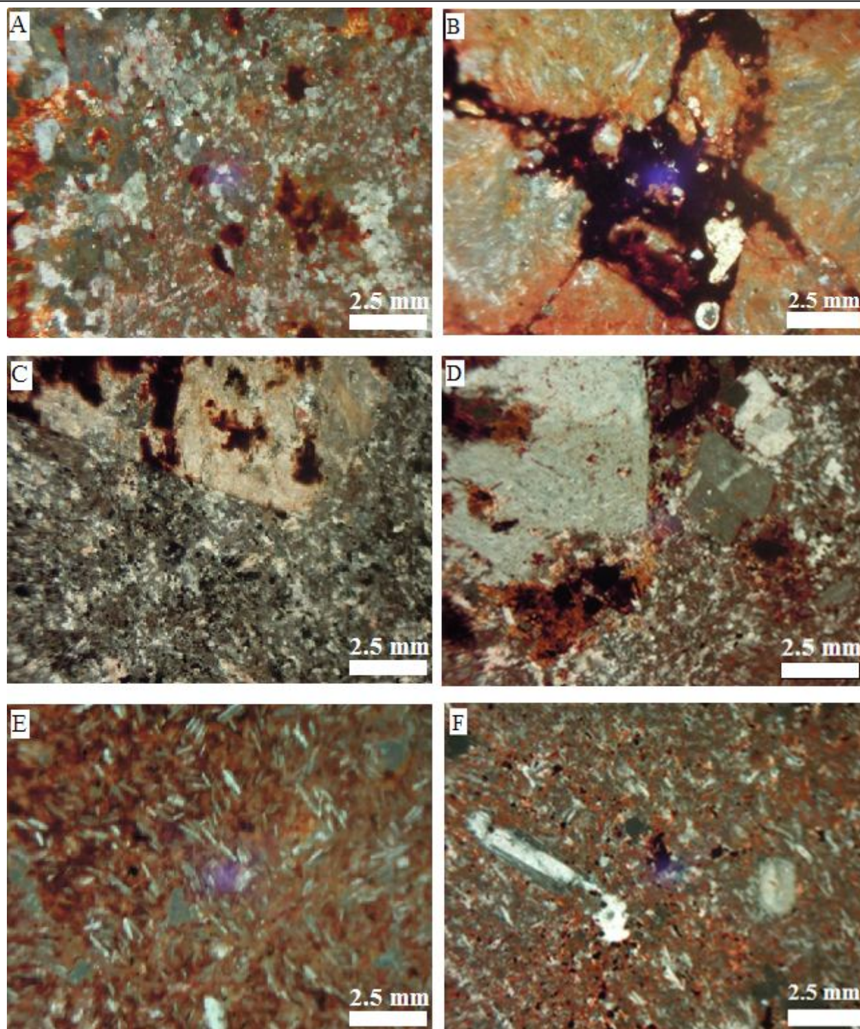
شکل ۴. انواع دگرسانی موجود در معدن فیروزه، A: دگرسانی سیلیسی در کوارتز تراکایت، B: دگرسانی سیلیسی ضعیف در برش با قطعات تراکیتی، C: دگرسانی آرژیلیکی با شدت متوسط در آندزیت، D: دگرسانی آرژیلیک با شدت ضعیف در آندزیت، E: دگرسانی آرژیلیک با شدت متوسط-سیلیسی در تراکیت و F: دگرسانی آرژیلیک با شدت ضعیف-سیلیسی در تراکی آندزیت
