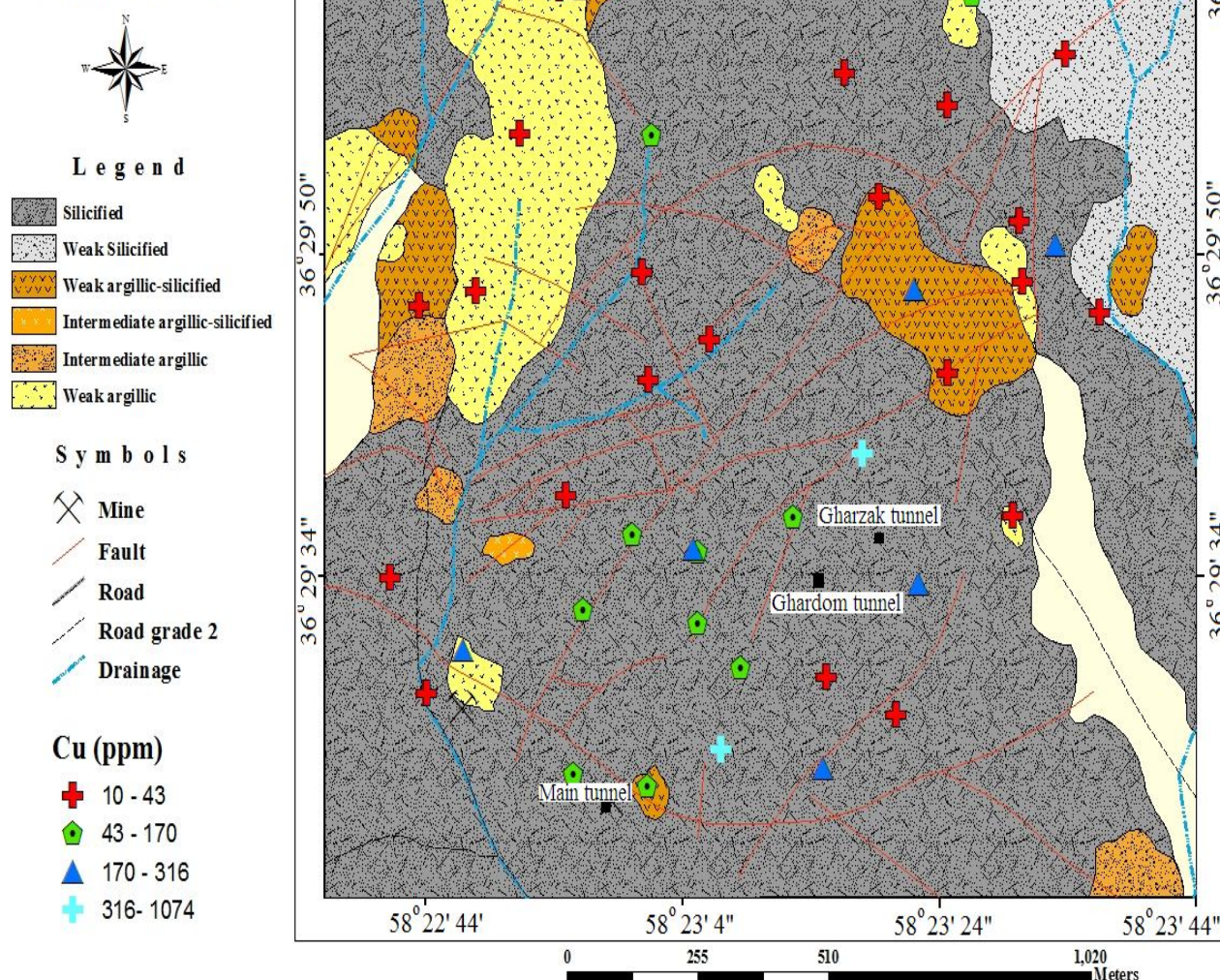
شکل ۱۱. نقشه پراکندگی عنصر مس در معدن فیروزه
