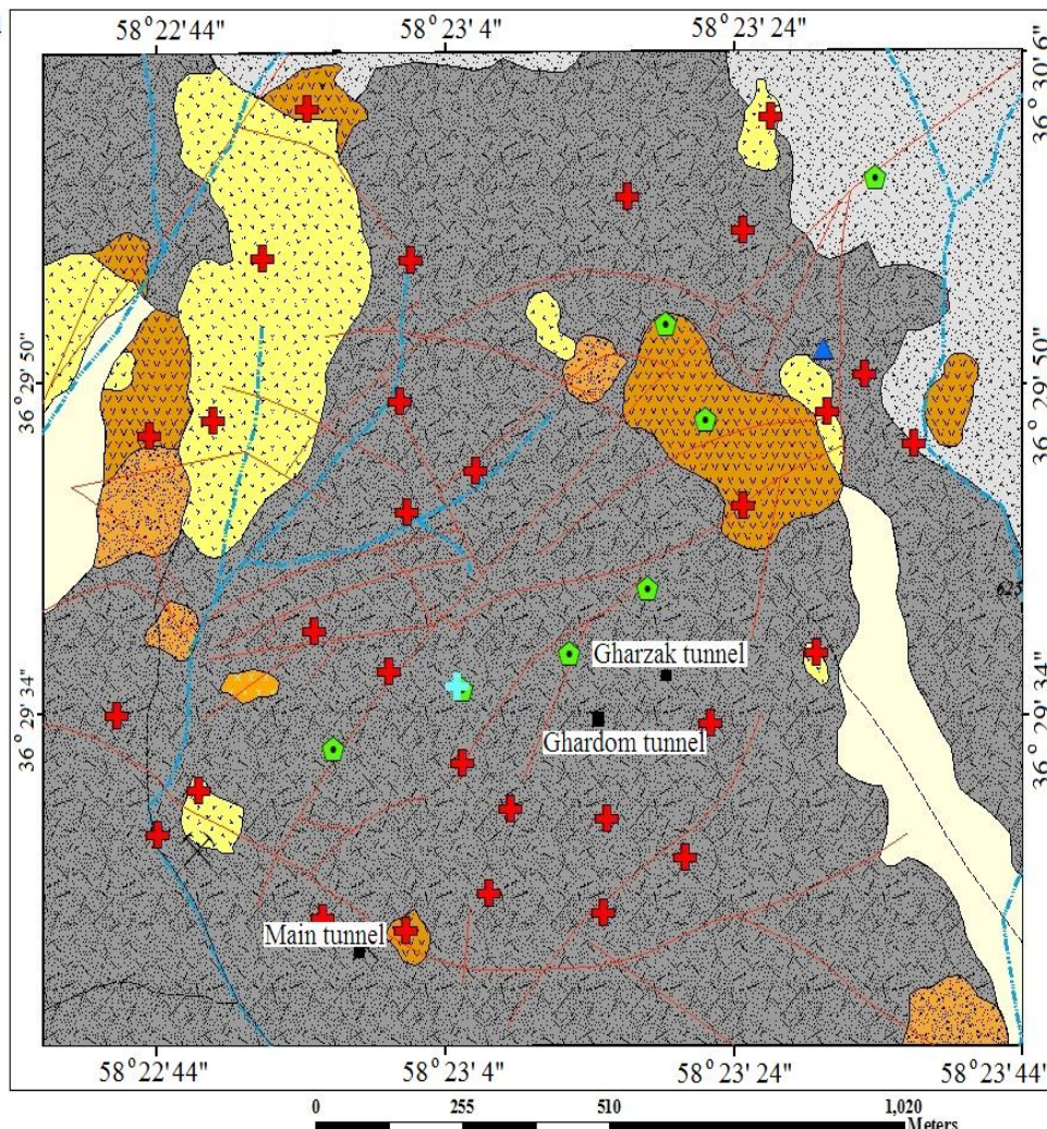
شکل ۱۰. نقشه پراکندگی عنصر طلا در معدن فیروزه
