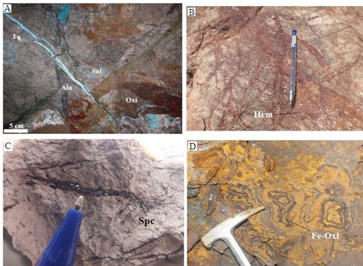
شکل ۶. تصاویر صحرایی از برخی کانی‌سازی‌ها و بافت و ساخت‌های موجود در معدن فیروزه. A: رگه‌چه‌های فیروزه و آلونیت کانی‌سازی‌های سولفیدی (پیریت، کالکوپیریت) و اکسیدی (هماتیت و مگنتیت) را قطع کرده است، B: برش هماتیتی، C: رگه-رگه‌های اسپکیولاریت در سنگ درون‌گیر تراکیت و D: وجود زوناسیون در هیدروکسید آهن، بیانگر وجود پیریت است. Tq: فیروزه، Sul: سولفید، Alu: آلونیت، Oxi: اکسید، Spc: اسپکیولاریت، Fe-Oxi: اکسیدهای آهن، Hem: هماتیت. علایم اختصاری بر اساس ویتنی و اوانز (Whitney and Evans, 2010)
