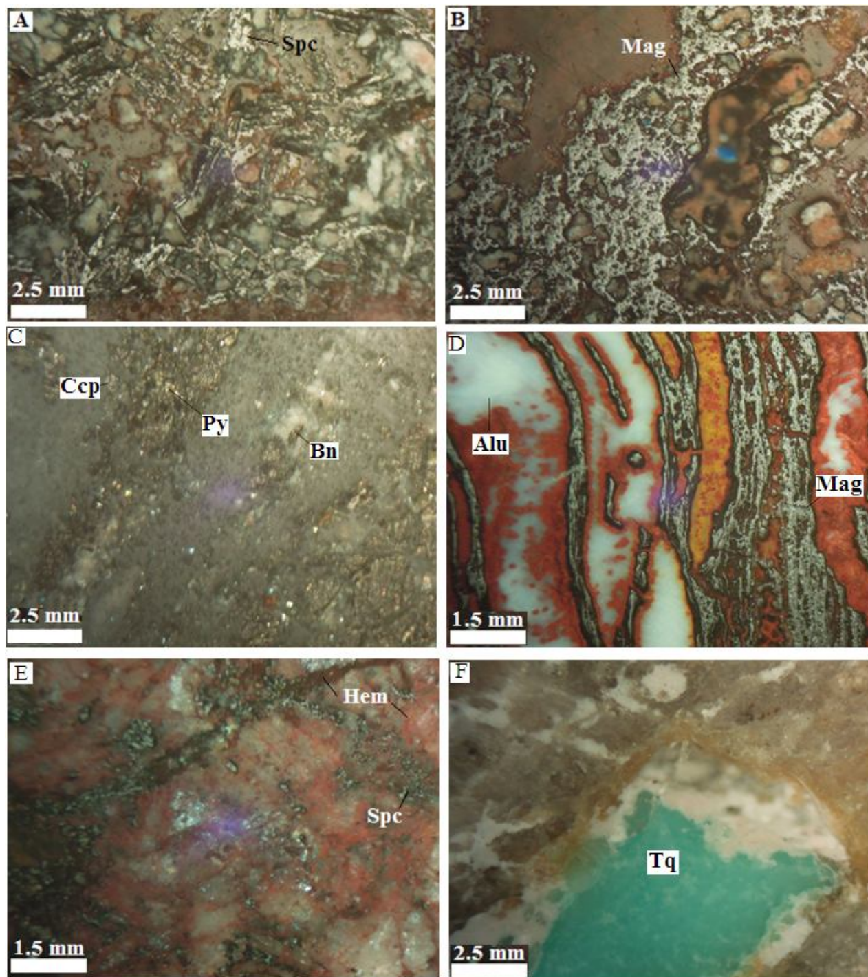
شکل ۷. تصاویر برخی از کانی‌های موجود در ماده معدنی در معدن فیروزه، A: رگچه‌های اسپکیولاریت، B: رگچه مگنتیت در زمینه‌ای برشی، C: دانه‌های پراکنده پیریت، کالکوپیریت و بورنیت، D: رگچه آلونیتی، E: رگچه اسپکیولاریت-هماتیت و F: فیروزه با بافت کلوئیدی. Spc: اسپکیولاریت، Mag: مگنتیت، Ccp: کالکوپیریت، Py: پیریت، Bn: بورنیت، Alu: آلونیت، Hem: هماتیت، Tq: فیروزه. علائم اختصاری بر اساس ویتنی و اوانز (Whitney and Evans, 2010)
