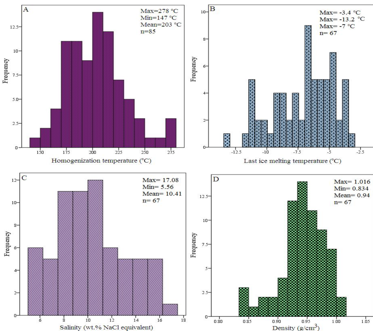
شکل ۱۲. نمودار فراوانی ریزدماسنجی برای سیالات درگیر معدن فیروزه، A: نمودار دمای همگن‌شدن، B: نمودار دمای ذوب یخ، C: نمودار شوری و D: نمودار چگالی
